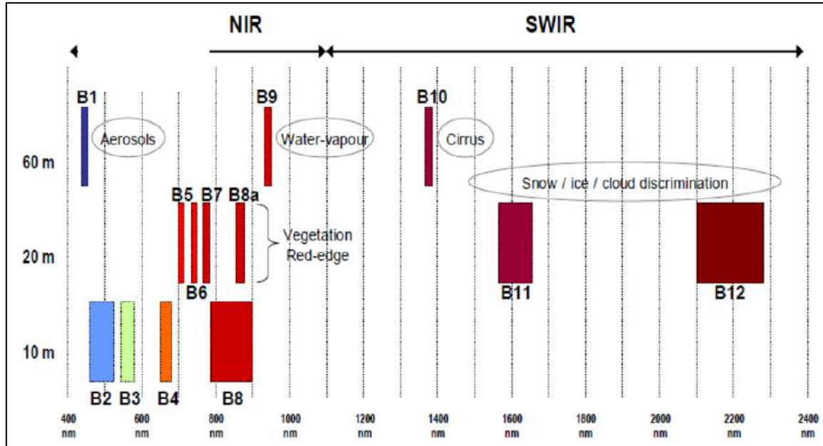
الشكل 1 : المتحسسات متعددة الاطيف مقابل دقة التمييز المكانية للمتحسسات التي يحملها القمر Sentinel2 (Gatti, and Galoppo, 2018).
