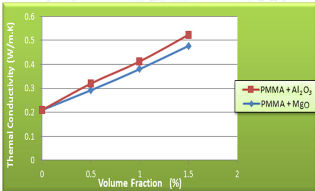
شكل (5) التوصيلية الحرارية كدالة للكسر الحجمي لدقائق أوكسيد الألمنيوم وأوكسيد المغنيسيوم النانوية لمادة مترابطة ذات أساس من البولي ميثا اكريليت
