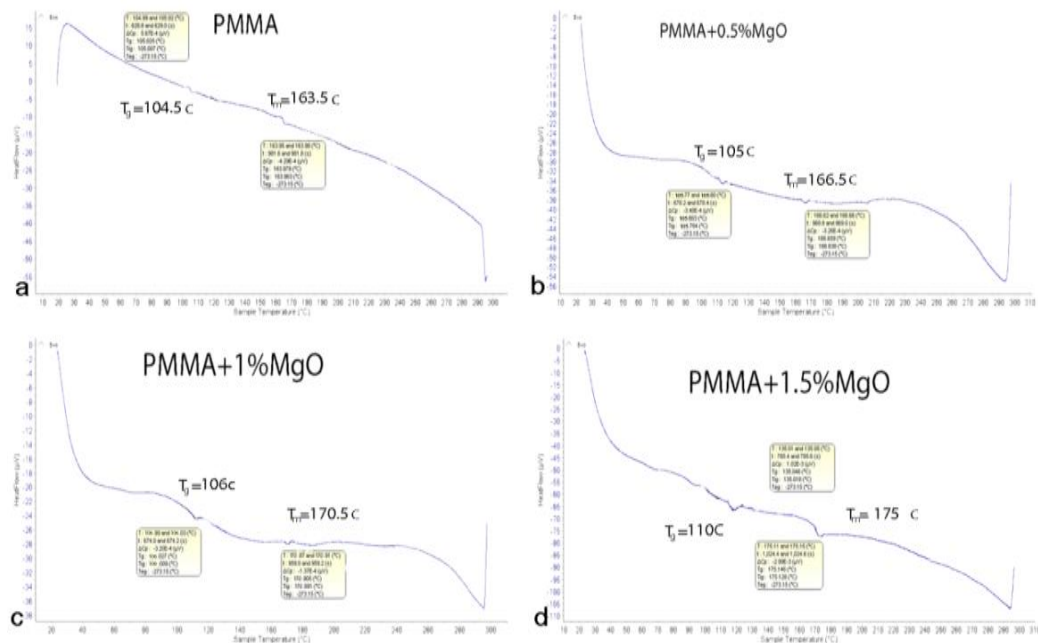
شكل (3) درجة حرارة إنتقال الزجاج وإنصهارها لمادة مترابطة ذات أساس بولي ميثا اكريليت المقواة بكسور حجمية مختلفة من دقائق أكسيد المغنيسيوم النانوية
