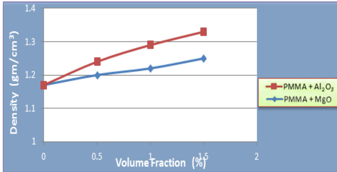
شكل (4) كثافة المادة المترابطة كدالة للكسر الحجمي لدقائق أوكسيد الألمنيوم وأوكسيد المغنيسيوم النانوية لمادة مترابطة ذات أساس من البولي ميثا اكريليت
