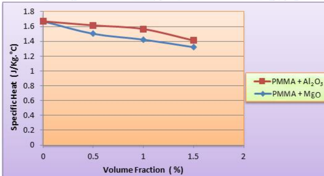
شكل (7) الحرارة النوعية كدالة للكسر الحجمي لدقائق أكسيد الألمنيوم وأكسيد المغنيسيوم النانوية لمادة مترابطة ذات أساس من البولي مثيل ميثا اكريليت
