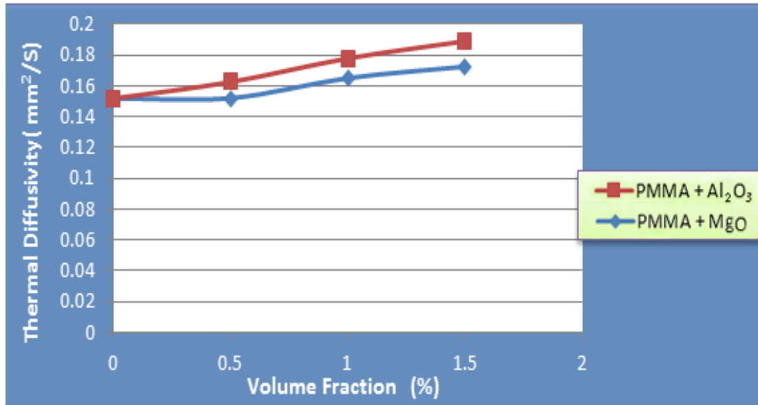
الشكل (6) الإنتشار الحراري كدالة للكسر الحجمي لدقائق أكسيد الألمنيوم وأكسيد المغنيسيوم النانوية لمادة مترابطة ذات أساس من البولي مثيل ميثا اكريليت
