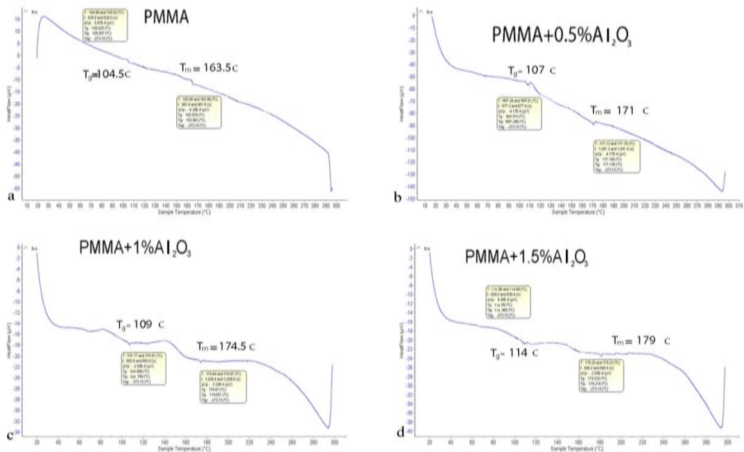
شكل (2) درجة حرارة إنتقال الزجاج وإنصهارها لمادة مترابطة ذات أساس من البولي ميثا اكريليت المقواة بكسور حجمية مختلفة من دقائق أكسيد الألمنيوم النانوية
