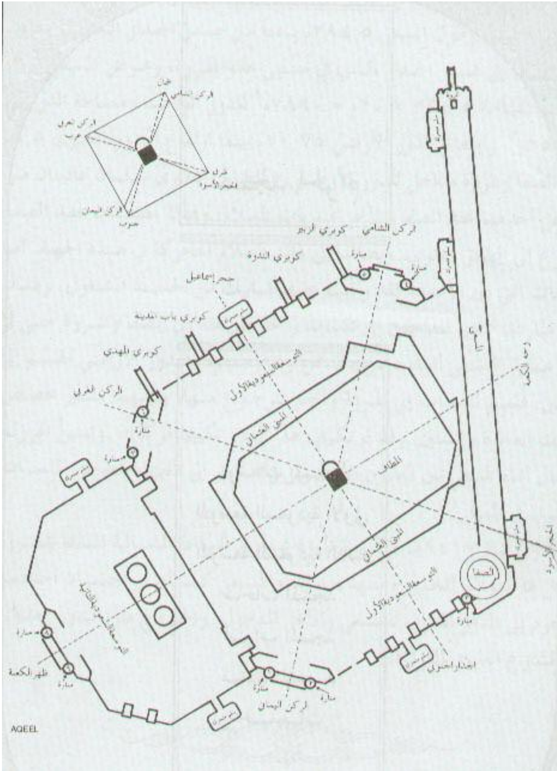
(شكل رقم ٩) مخطط عام للحرم المكي الحديث يوضح فيه موقع الكعبة والتوسعات الجديدة وبظمنها مضمار الصفا والمروة المصدر :- دائرة الحرم الشريف
