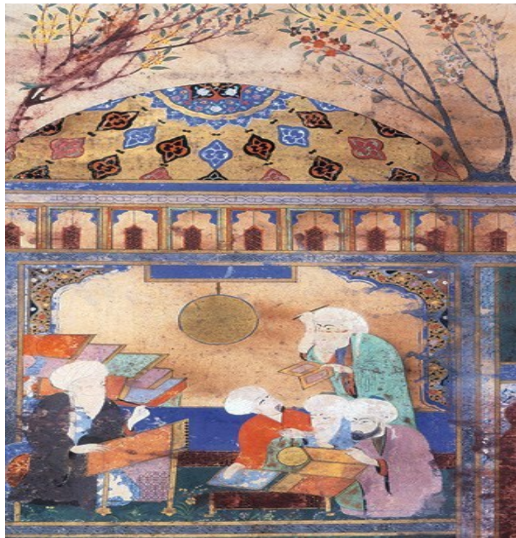
المنمنمة ١ / نصير الدين الطوسي في مرصده الفلكي / المتحف البريطاني - لندن https://Nasir_al-Din_al-Tusi_at_observatory.jpg
