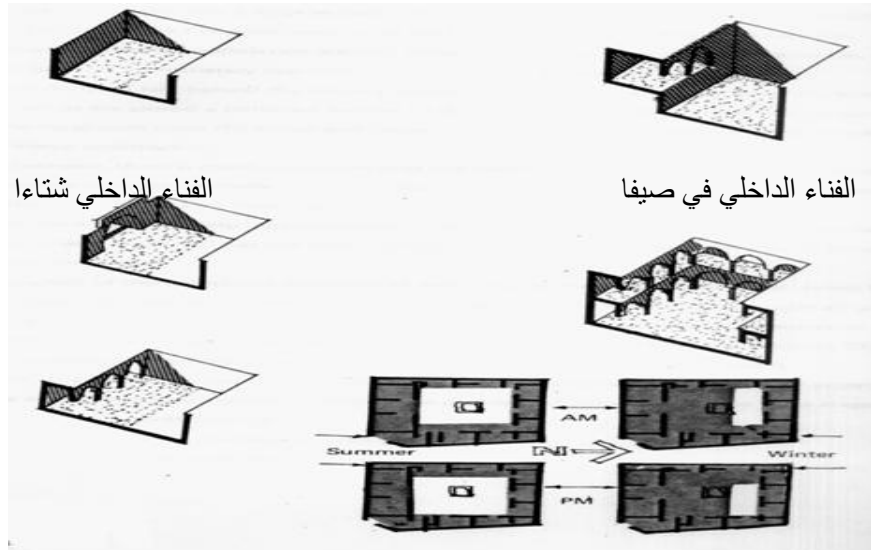
شكل (5) البيت البغدادي التقليدي وتغيراته خلال مراحل السنة بين الصيف والشتاء وتأثير الظل والضوء عليه.
