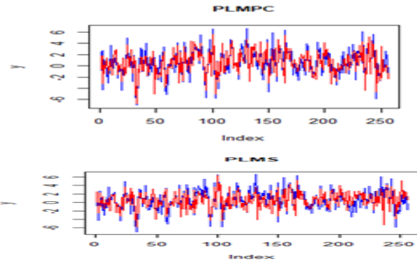
الشكل رقم (2-3) اعلاه يمثل قيم عندما \sigma_e = 1 و حجم العينة ( n=256 ) و عدد المتغيرات تساوي ( ثمانية متغيرات ) باستخدام المعادلة M1
