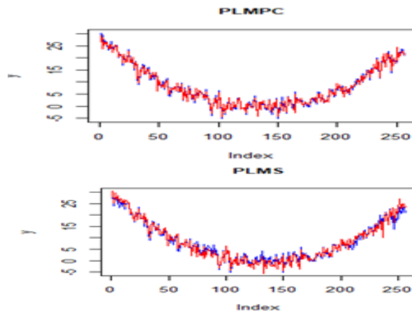
الشكل رقم (3-3) اعلاه يمثل قيم عندما \sigma_e = 2 و حجم العينة ( n=256 ) و عدد المتغيرات تساوي ( ثمانية متغيرات ) باستخدام المعادلة M1
