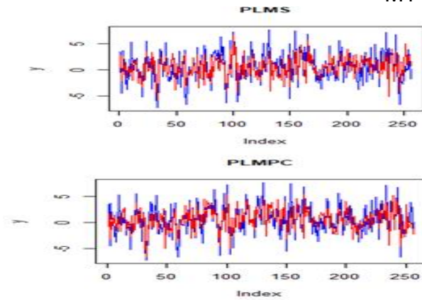
الشكل رقم (3-3) اعلاه يمثل قيم عندما \sigma_e = 2 و حجم العينة ( n=256 ) و عدد المتغيرات تساوي ( ثمانية متغيرات ) باستخدام المعادلة M1
