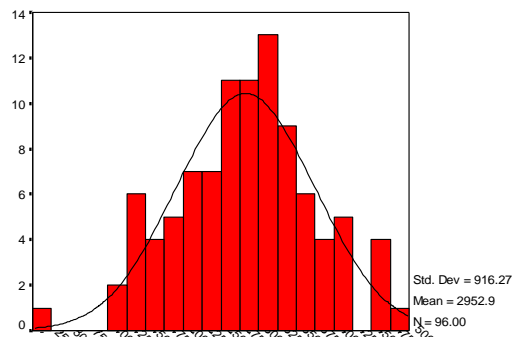
الشكل رقم (3) يوضح توزيع المتغير المعتمد (عدد النباتات) على وفق التوزيع الطبيعي
