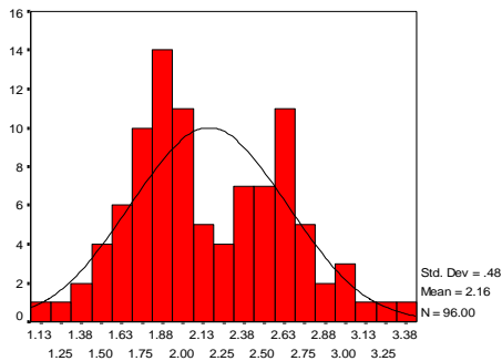
الشكل رقم (2) يوضح توزيع المتغير (طن/هـ) على وفق التوزيع الطبيعي
