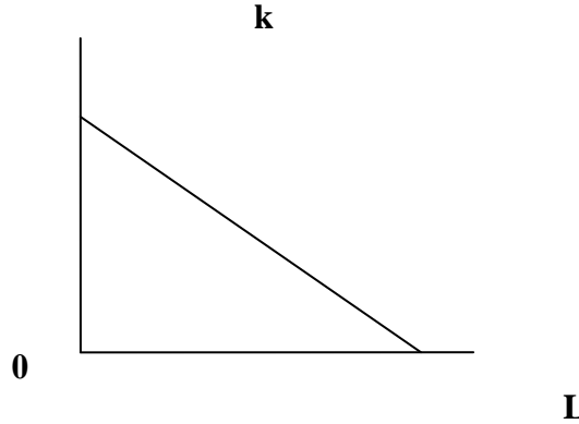
شكل (1) الدالة الخطية
