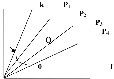
شكل (3) دالة البرمجة الخطية
