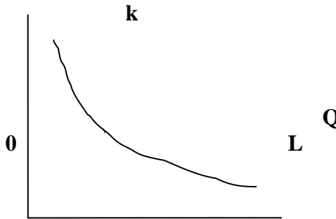
شكل (4) دالة الناتج المحدب
