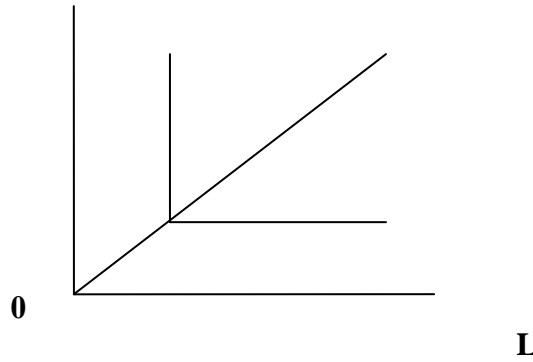
شكل (2) دالة المدخل والمنتج
