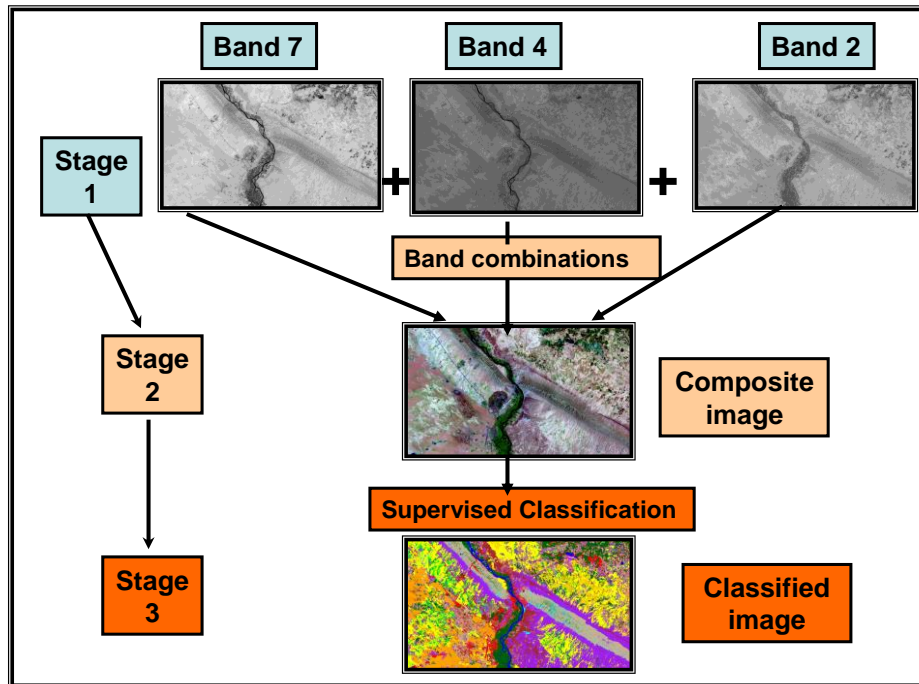
الشكل - 4: المرئية الفضائية المركبة من القنوات (2،4،7) من القمر لاندسات للعام 2006 لمنطقة بيجي شمال العراق.
