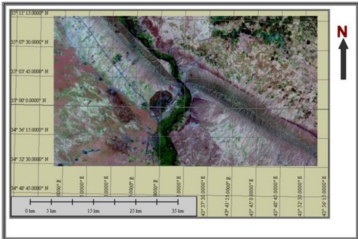
الشكل 4: المرئية الفضائية المركبة من القنوات (2،4،7) من القمر لاندسات للعام 2006 لمنطقة بيجي شمال العراق.
