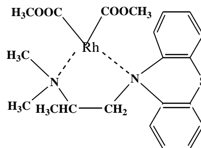
PRZH-Rh (II)
