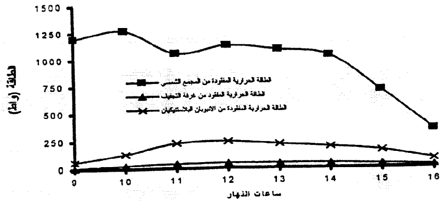
شكل (١): الطاقة الحرارية المفقودة من اجزاء المجفف الشمسي في فصل الصيف.
