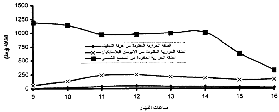
شكل (٢): الطاقة الحرارية المفقودة من اجزاء المجفف الشمسي في فصل الشتاء.
