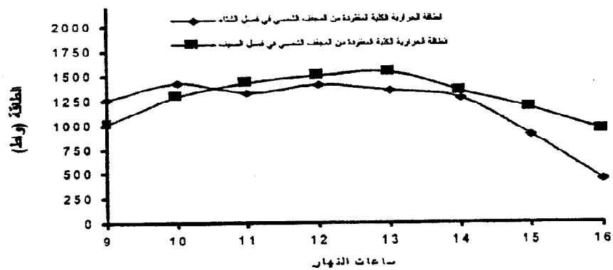
شكل (٣): الطاقة الحرارية المفقودة من المجفف الشمسي في فصلي الصيف والشتاء.
