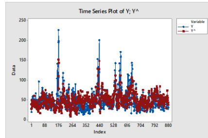
الشكل (5): التطابق بين البيانات الاصلية مع البيانات التقديرية (سلسلة التنبؤ ( PM_{10} ) خلال الفترة الكلية لبيانات الاختبار بطريقة MLR.
