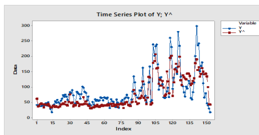
الشكل (9): التطابق بين البيانات الاصلية مع البيانات التقديرية (سلسلة التنبؤ) للمتغير المعتمد ( PM_{10} ) لبيانات الاختبار باستخدام RNN-Wavelet الهجينة.
