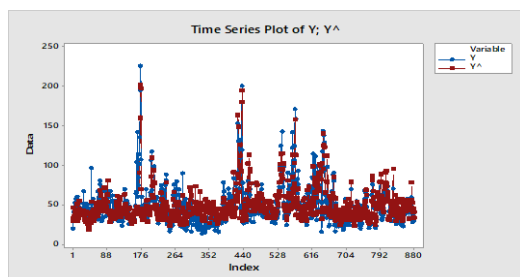
الشكل (6): التطابق بين البيانات الاصلية مع البيانات التقديرية (سلسلة التنبؤ) للمتغير المعتمد ( PM_{10} ) خلال الفترة الكلية لبيانات التدريب باستخدام MLR-RNN.
