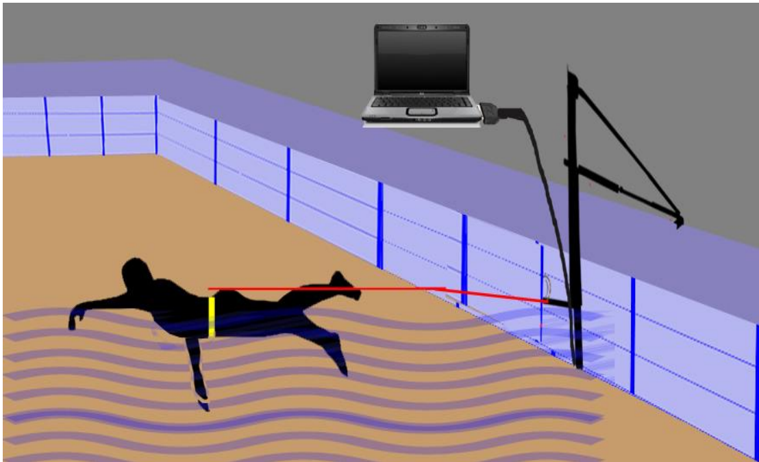
الشكل (١) يوضح اجزاء الجهاز المستخدم لقياس القوة الدافعة للسباحين وطريقة استخدامه مع جسم السباح.
