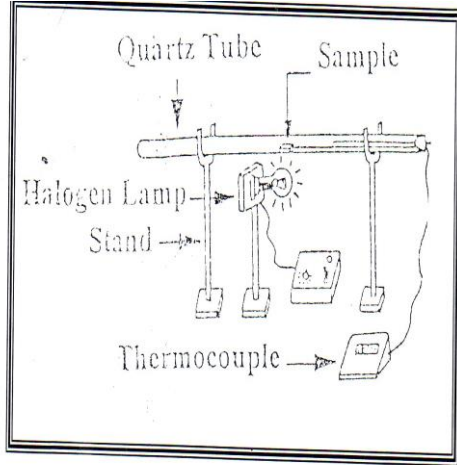
شكل (1) يوضح منظومة التلدين الايزوثيرمي السريع
