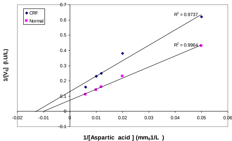
شكل رقم(3): رسم لنينوفر-بيرك لحساب ثابت ميكالس-منتن للمتئاظر II المنقى من إدرار الأصحاء والمرضى المصابين بـ (CRF)
