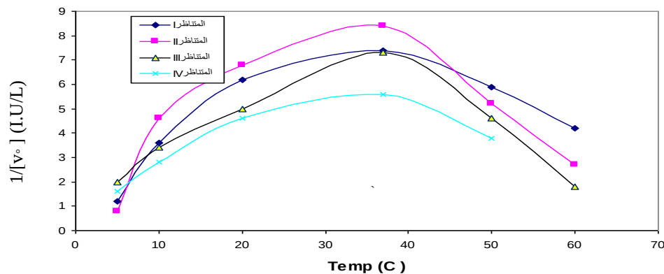
شكل رقم (7): تأثير درجة الحرارة في سرعة تفاعل المتناظرات I, II, III, IV
