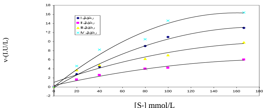
شكل رقم (1): العلاقة بين تراكيز مختلفة من (حامض الاسبارتيك) ملي مول /لتر وسرعة تفاعل المتناظرات I, II, III, IV المنقاة من إدرار المرضى المصابين بـ (CRF).
