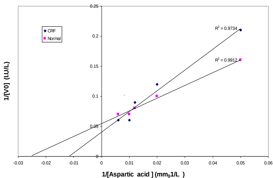
شكل رقم (5): رسم لنيوفر-بيرك لحساب ثابت ميكالس-منتن للمتناظر IV المنقى من إدرار الأصحاء والمرضى المصابين بـ (CRF)
