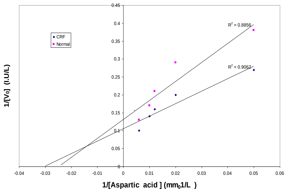
شكل رقم (4): رسم لنيوفر-بيرك لحساب ثابت ميكالس-منتن للمتناظر III المنقى من إدرار الأصحاء والمرضى المصابين بـ (CRF)
