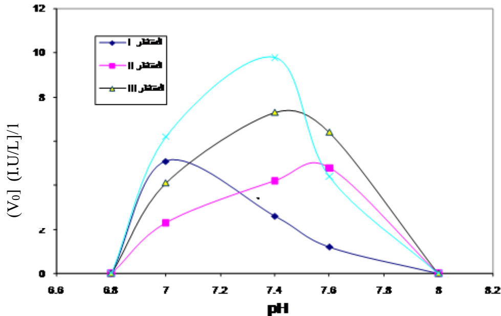
شكل رقم (6): تأثير الأس الهيدروجيني على سرعة تفاعل المتناظرات I, II, III, IV المنقاة من ادرار المرضى المصابين بـ (CRF).
