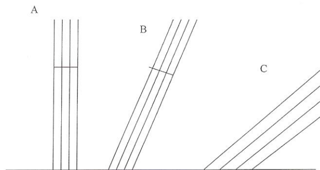
شكل (3) علاقة زاوية الشمس مع فاعلية الأشعة الشمسية . A الشمس عمودية مباشرة فاعلية للغة B زاوية سقوط أصغر اشعاع شمسي أقل فاعلية في كل وحدة مساحة . B زاويا سقوط أصغر بكثير اشعاع شمسي خفيف في كل وحدة مساحة .
