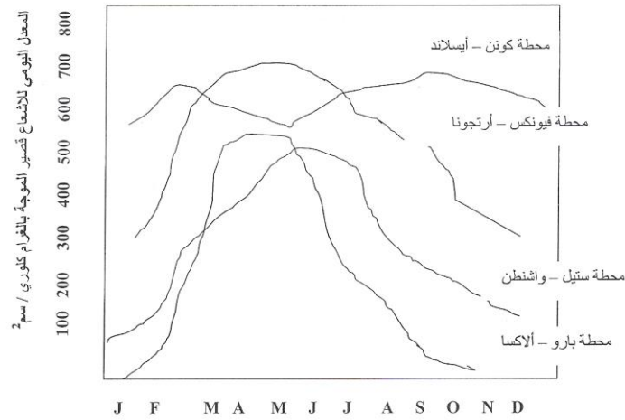
شكل رقم 2 التقدم السنوي في متوسط الأشعاع الشمسي عند محطات معينة
