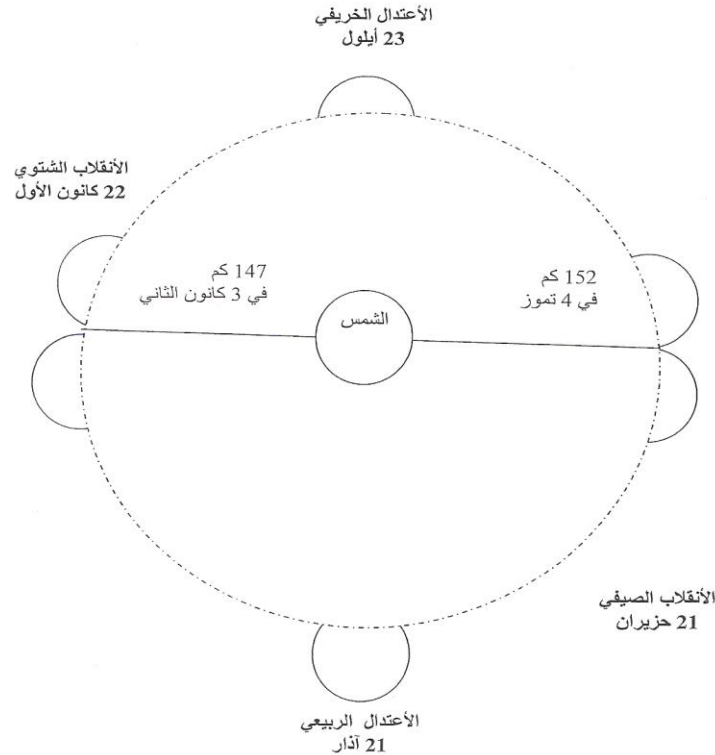
شكل رقم (1) مدار الأرض حول الشمس
