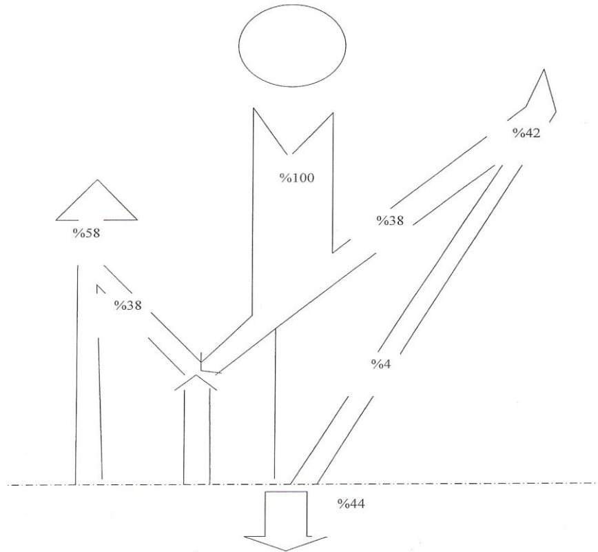
شكل رقم (4) يوضح الموازنة الإشعاعية للكرة الأرضية
