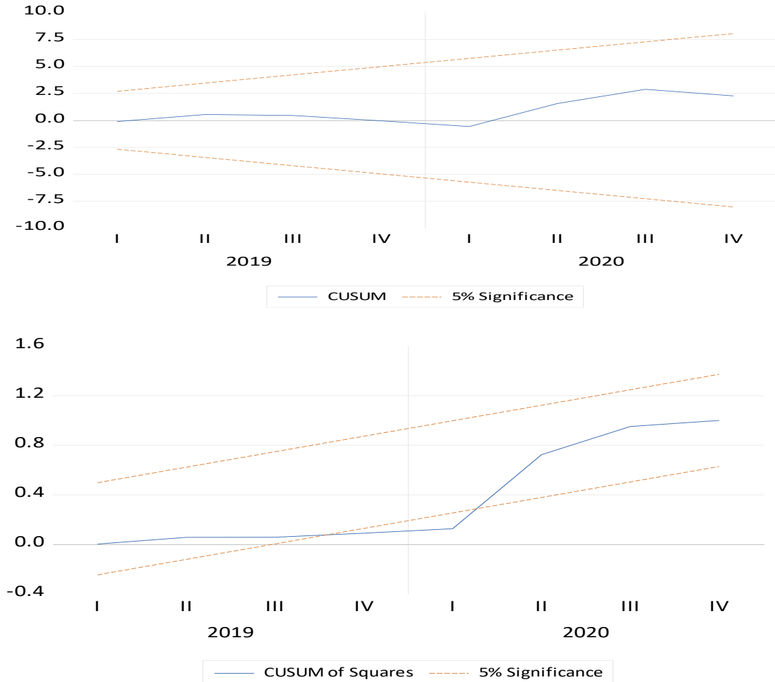
شكل (٣): اختبار الاستقرار الهيكلي لمعاملات النموذج
