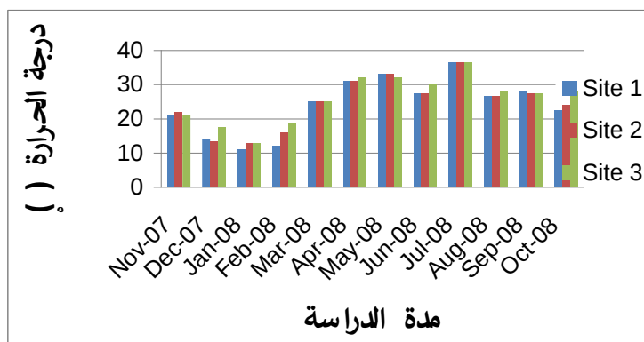
شكل (2) درجة حرارة الهواء في المواقع الثلاثة خلال مدة الدراسة.
