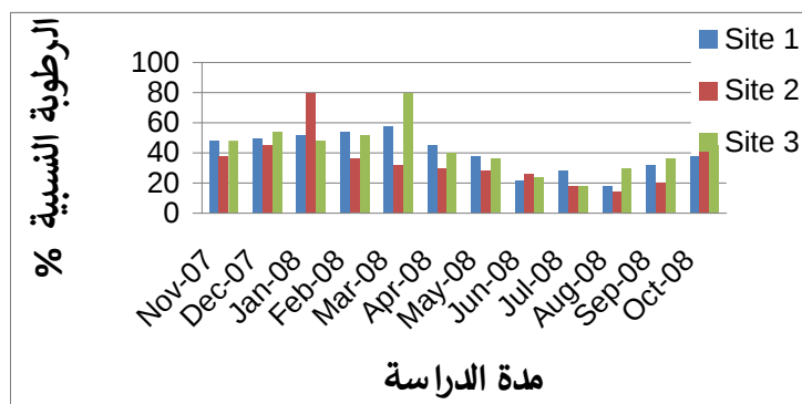
شكل (4) الرطوبة النسبية للتربة في المواقع الثلاثة خلال مدة الدراسة.
