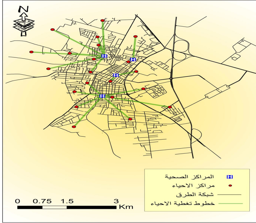
الشكل ٨. نموذج تحليل تخصيص الموقع للمراكز الصحية في مدينة المفرق.
