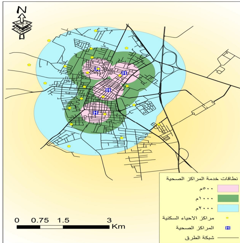
الشكل ٩. النطاقات المتعددة لخدمة المراكز الصحية في مدينة المفروق.
