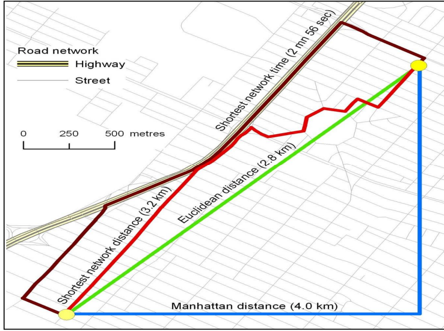
الشكل ٥. طرق التعبير عن المسافة. المصدر: (Apparicio, P. 2003)
