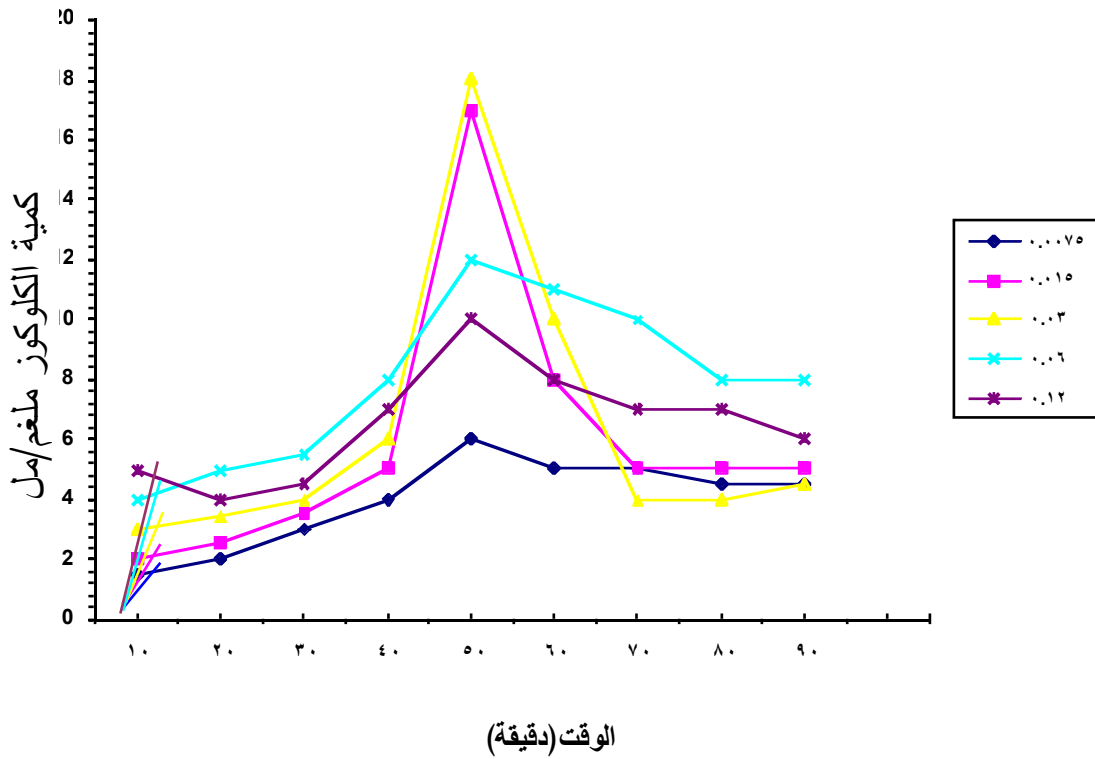
شكل (a3): تأثير تركيز الكلوكواميليز في تحليل نشا الذرة الخام 2A % (v/w) في pH (4.2) ودرجة 40 °م.
