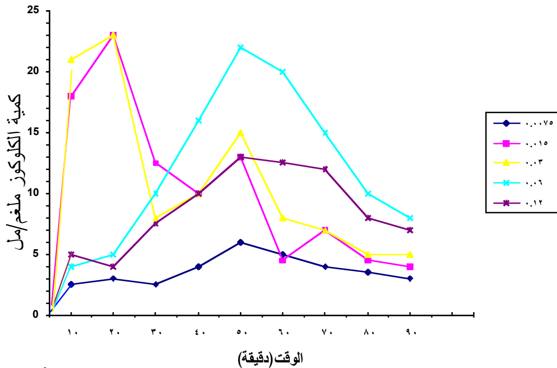
شكل (b3): تأثير تركيز الكلوكواميليز في تحليل نشا البطاطا الخام 2B % (v/w) في pH (4.2) ودرجة 40 °م
