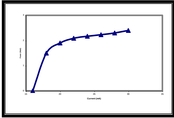
شكل (٤) تغير قدرة الخرج الليزري مع تيار التفريغ الكهربائي.
