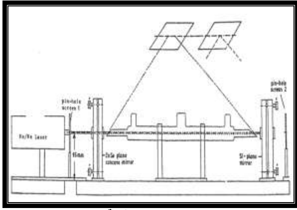
شكل (2) يوضح اجراء الترصيف لمنظومة ثاني اوكسيد الكربون المستمر.
