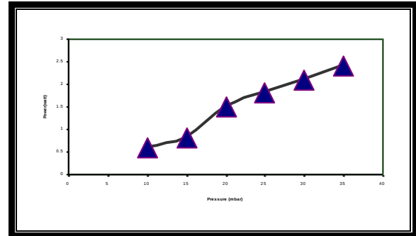
شكل (٣) تغير قدرة الخرج الليزري مع ضغط الغاز.
