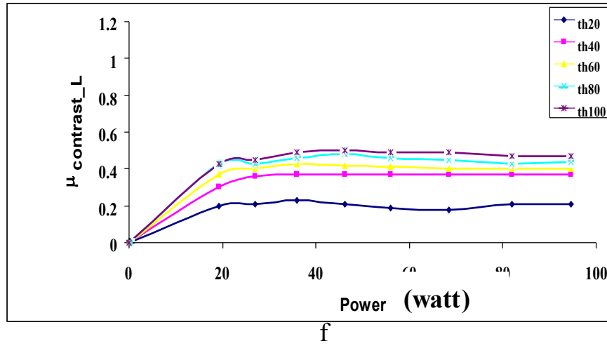
شكل ( 13 ) تقنيات التباين للصورة الاختبارية مصدر الإضاءة مصباح التلكنستن لقيم عتبات ( th )
