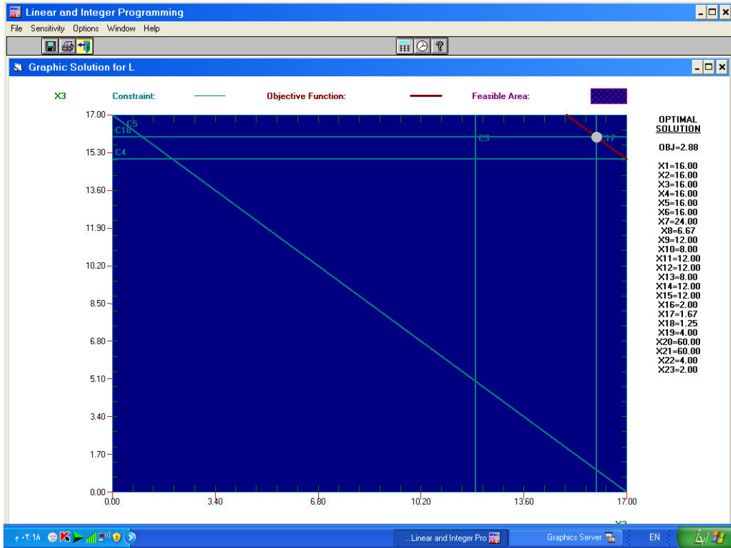
الشكل رقم (١) الحل الأمثل بواسطة طريقة الخطوط البيانية
