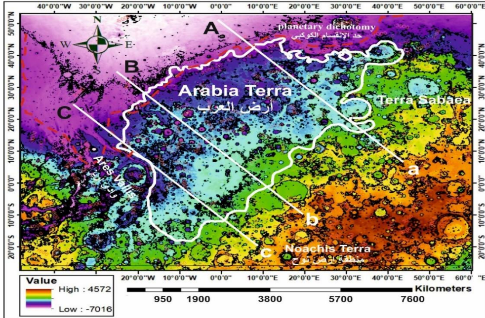
الشكل (٥) خارطة طبوغرافية منطقة أرض العرب - Arabia Terra
