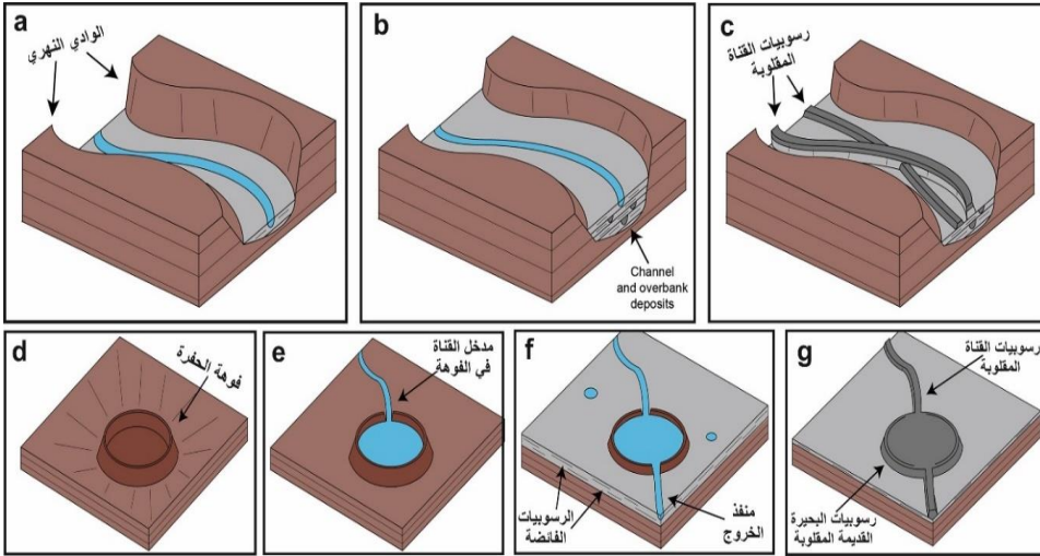
الشكل (٨) مخطط يوضح التطور المفسر لشبكات الوادي المملوءة جزئياً (a - c), و (d - g) رواسب البحيرات القديمة المقلوبة, وفقاً لـ (Cardenas et al., 2017; Davis et al., 2019)
