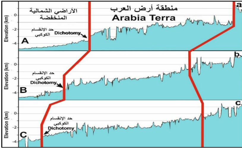
الشكل (٦) المقاطع الطبوغرافية لمنطقة (أرض العرب - المحددة ضمن الخطوط الحمراء) بحسب ترتيبها في (الشكل ٥)، المخطط بتصرف عن (Zachary, 2022; MOLA topography data).
