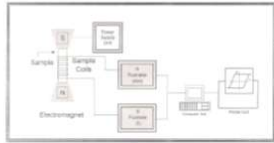
شكل (1) المخطط التصيلي لمتابعة اختبار الخاص المغناطيسية
