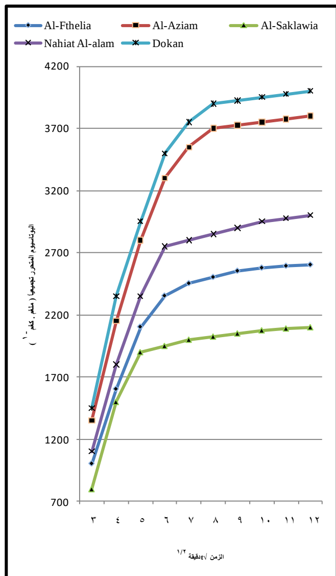
شكل (3) : منحنيات العلاقة بين مؤشر كمية البوتاسيوم المتحررة والزمن لتحديد مسار التفاعل الكيميائي لعملية التححرر
