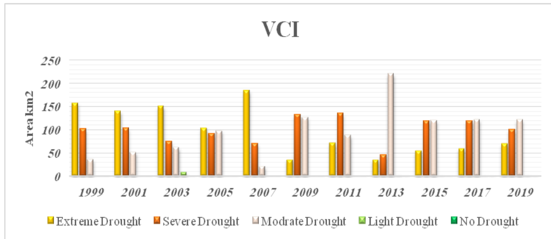
شكل 5. التوزيع البياني لمساحات منطقة الدراسة حسب دليل الجفاف VCI.
