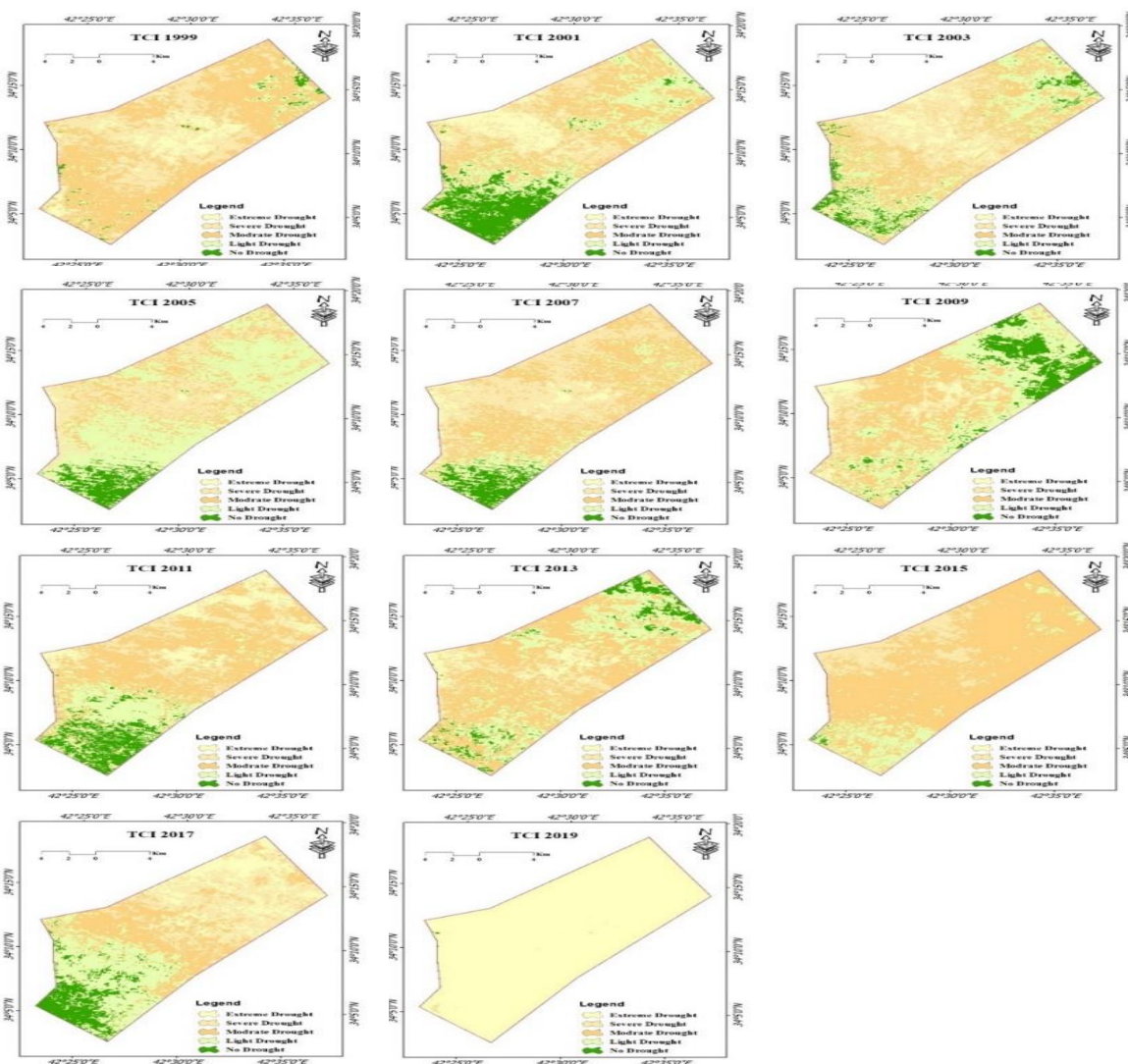
شكل 8. خرائط المنطقة حسب دليل الجفاف TCI للمنطقة خلال مدة الواسعة 1999-2019.
