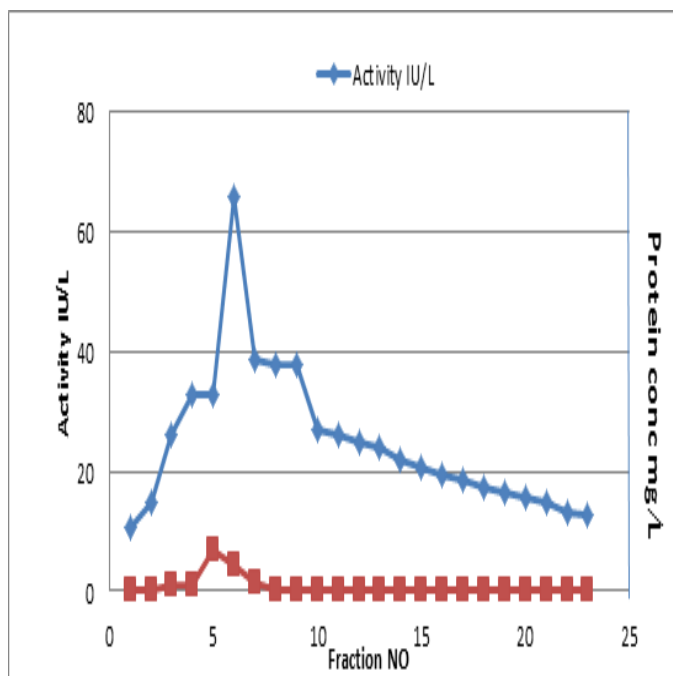
الشكل (١) تنقية ALP بواسطة كروماتوغرافيا الترشيح الهلامي
