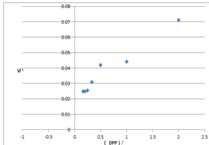
الشكل (٣) رسم لينوفر - برك لحساب قيمة Km و Vmax
