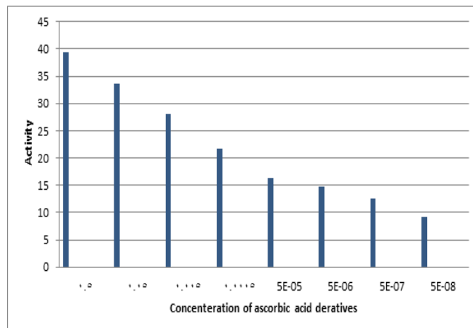
الشكل (٧) تأثير بعض مشتقات حامض الاسكوربيك على فعالية انزيم
