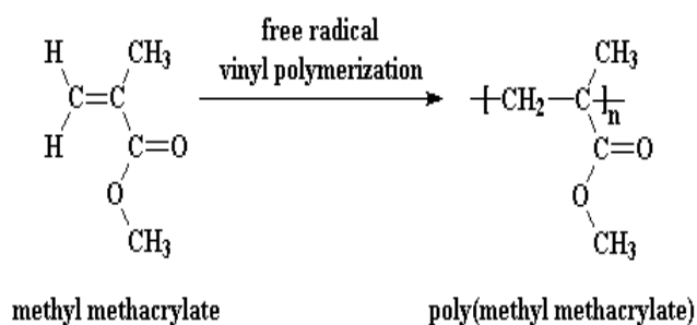
شكل (1) معادلة بلمرة الـ (PMMA)
