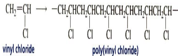
شكل (3) معادلة بلمرة متعدد (كلوريد الفينيل)
