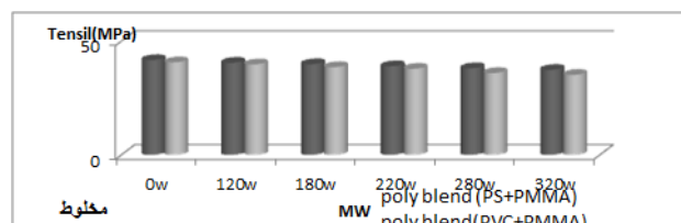
شكل (4) قيم اختبار إجهاد الشد قبل وبعد التشيع (المتجانسة و المشتركة و المخلوطة)
