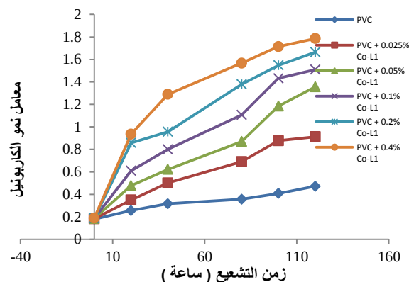
الشكل (١٥): العلاقة بين معامل امتصاص الكاربونيل وزمن التشعيع لرقبة متعدد (كلوريد الفينيل) النقية والرقائق المحتوية على تراكيز مختلفة من المعقد Co-L1
