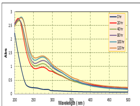
الشكل (٦): التغير في طيف الاشعة فوق البنفسجية - المرئية لمتعدد (كلوريد الفينيل) المحتوية على تركيز ٠.٤ % من المعقد ( Co-L1 ) بسمك (70±5) مايكرون عند ازمان التشعيع
