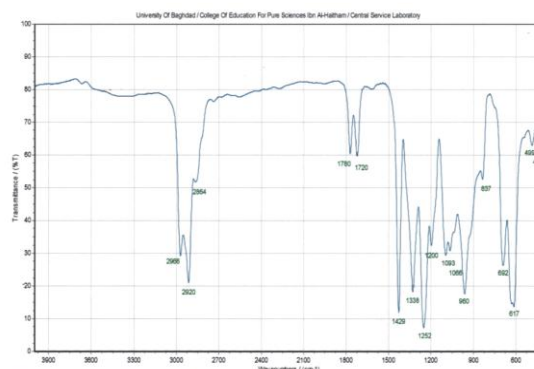
شكل (١٢): طيف الاشعة تحت الحمراء لرقائق متعدد (كلوريد الفينيل) النقية قبل التشيع
