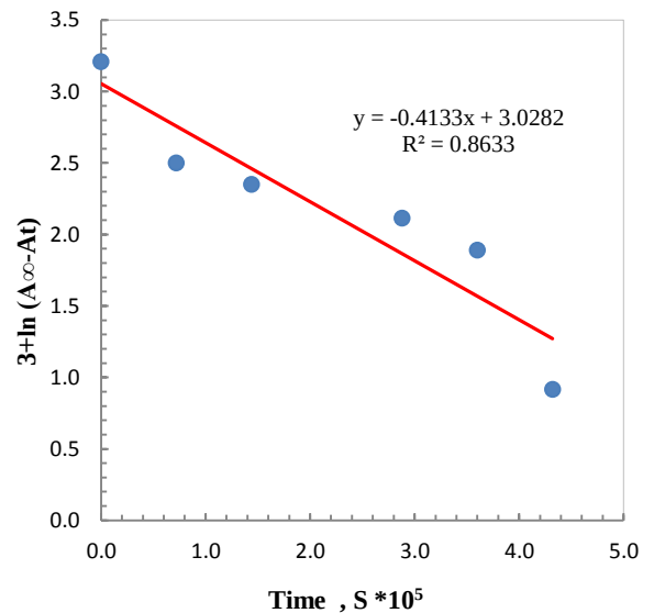
الشكل (٧) : العلاقة بين اللوغاريتم الطبيعي لامتناسية المعدن (Co-L1) بتركيز ٠.٢٥% في رقائق متعدد (كلوريد الفينيل) ذات السمك (70±5) مايكرون مع زمن التشيع
