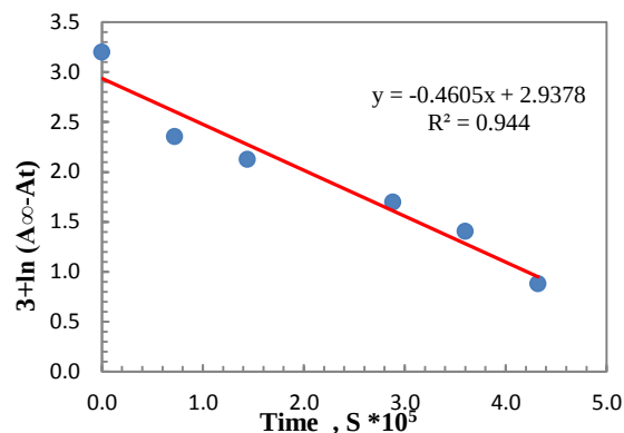
الشكل (١١): العلاقة بين اللوغاريتم الطبيعي لامتصاصية المعقد Co-L1 ( بتركيز ٠.٤ % في رقائق متعدد (كلوريد الفينيل) ذات السمك (70±5) مايكرون مع زمن التشيع
