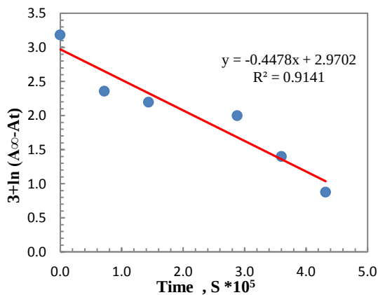
الشكل (١٠) : العلاقة بين اللوغاريتم الطبيعي لامتناسية المعدن (Co-L1) بتركيز ٠.٢% في رقائق متعدد (كلوريد الفينيل) ذات السمك (70±5) مايكرون مع زمن التشيع
