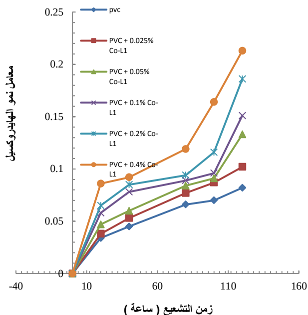
الشكل (١٦): العلاقة بين معامل امتصاص الكاربونيل I_{OH} وزمن التشعيع لرقبة متعدد (كلوريد الفينيل) النقية والرقائق المحتوية على تراكيز مختلفة من المعقد Co-L1
