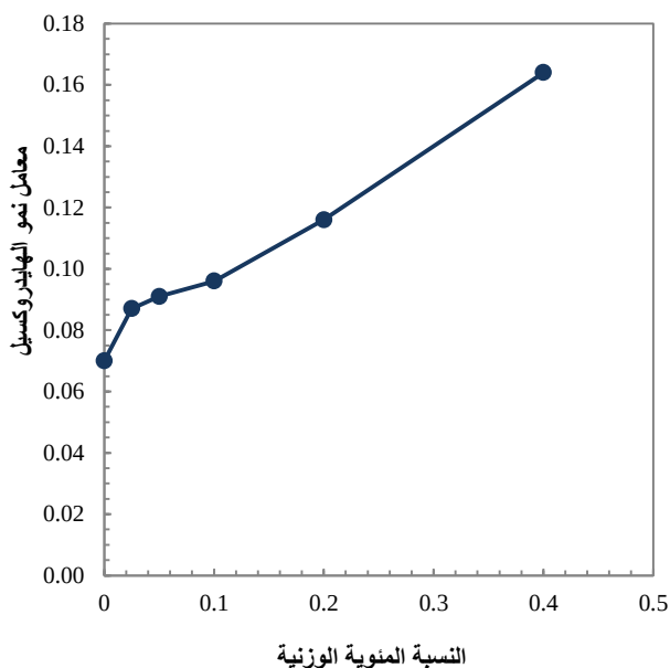
الشكل (١٨): التغير في معامل امتصاص الكاربونيل I_{OH} مع تركيز المعقد Co-L1 لرقائق متعدد (كلوريد الفينيل) ولزمن تشعيع ١٠٠ ساعة
