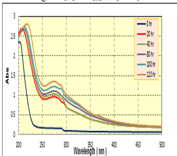
الشكل (٥): التغير في طيف الاشعة فوق البنفسجية - المرئية لمتعدد (كلوريد الفينيل) المحتوية على تركيز ٠.٢ % من المعقد ( Co-L1 ) بسمك (70±5) مايكرون عند ازمان التشعيع
