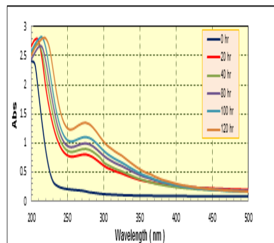
الشكل (٣): التغير في طيف الاشعة فوق البنفسجية - المرئية لمتعدد (كلوريد الفينيل) المحتوية على تركيز ٠.٥ % من المعقد ( Co-L1 ) بسمك (70±5) مايكرون عند ازمان التشعيع
