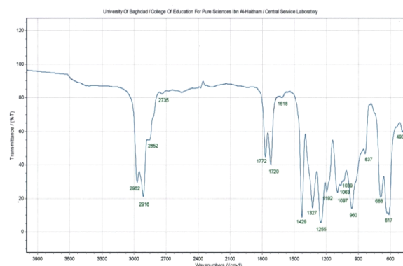
الشكل (١٣): طيف الاشعة تحت الحمراء لرقائق متعدد (كلوريد الفينيل) النقية بعد ١٢٠ ساعة التشيع
