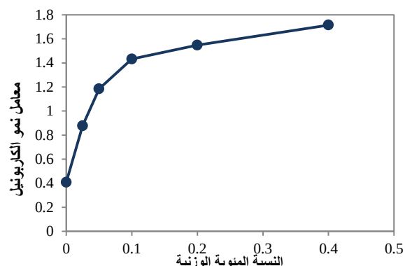
الشكل (١٧): التغير في معامل امتصاص الكاربونيل I_{Co} مع تركيز المعقد Co-L1 لرقائق متعدد (كلوريد الفينيل) ولزمن تشعيع ١٠٠ ساعة
