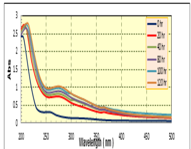
الشكل (٢): التغير في طيف الاشعة فوق البنفسجية - المرئية لمتعدد (كلوريد الفينيل) المحتوية على تركيز ٠.٢٥ % من المعقد ( Co-L1 ) بسمك (70±5) مايكرون عند ازمان التشعيع
