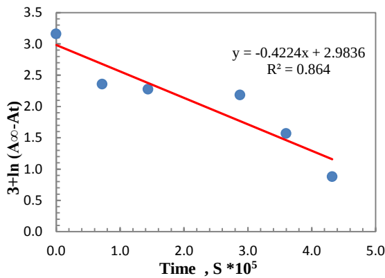
الشكل (٩) : العلاقة بين اللوغاريتم الطبيعي لامتناسية المعدن (Co-L1) بتركيز ٠.١% في رقائق متعدد (كلوريد الفينيل) ذات السمك (70±5) مايكرون مع زمن التشيع
