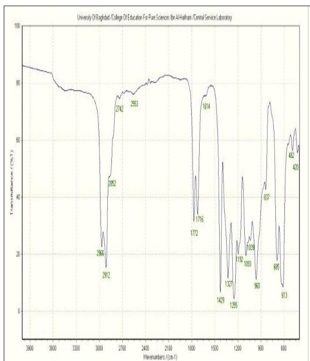
الشكل (١٤): طيف الاشعة تحت الحمراء لرقائق متعدد (كلوريد الفينيل) المحتوية على تركيز ٠.٤ % من المعقد Co-L1 بعد ١٢٠ ساعة تشيع
