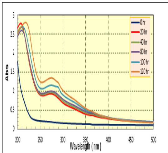
الشكل (٤): التغير في طيف الاشعة فوق البنفسجية - المرئية لمتعدد (كلوريد الفينيل) المحتوية على تركيز ٠.١ % من المعقد ( Co-L1 ) بسمك (70±5) مايكرون عند ازمان التشعيع
