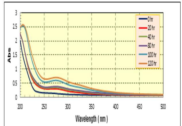
الشكل (١): التغير في طيف الاشعة فوق البنفسجية - المرئية لمتعدد (كلوريد الفينيل) الخالي من المضافات بسمك (70±5) مايكرون عند ازمان التشعيع
