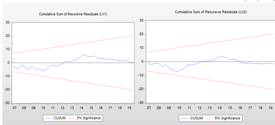
الشكل (٤): الرسم البياني لأختبار (CUSUM).
