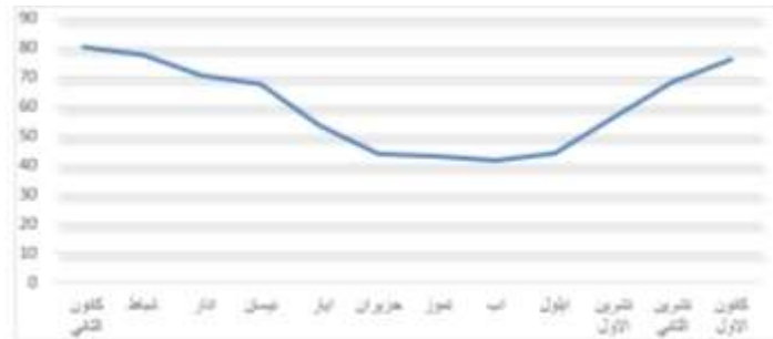
الشكل (٤) معدل الرطوبة النسبية السنوية لمحطة حبات للمدة (٢٠٠٢-٢٠٢٢)
