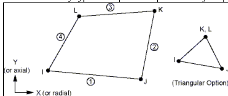
Fig.(16) Fluid141 element
