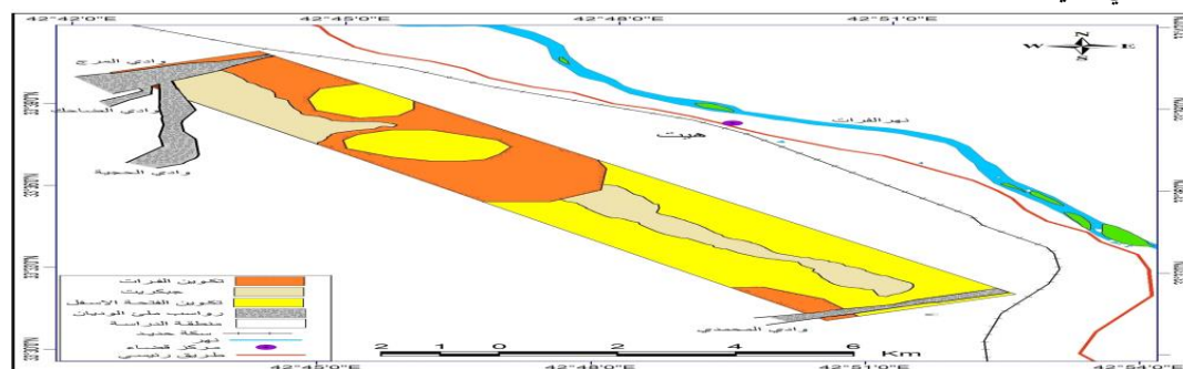
شكل 3. الخارطة الجيولوجية لمنطقة الدراسة المصدر (Geological Heat Plate، 2000) مقياس 1:25000 لسنة 2000، وبرنامج GIS 10.6
