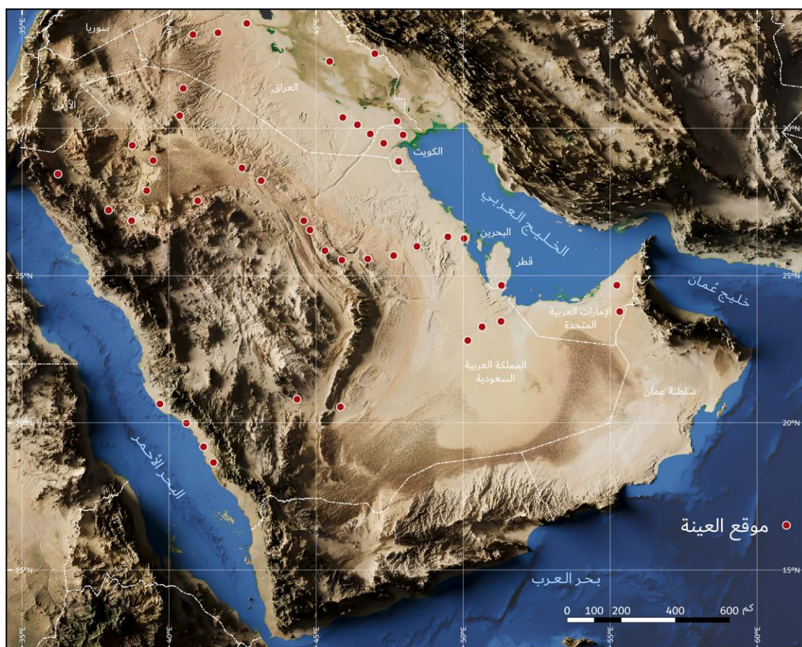
شكل 2. مواقع أخذ العينات للكتبان الرملية في الشرق الأوسط.
