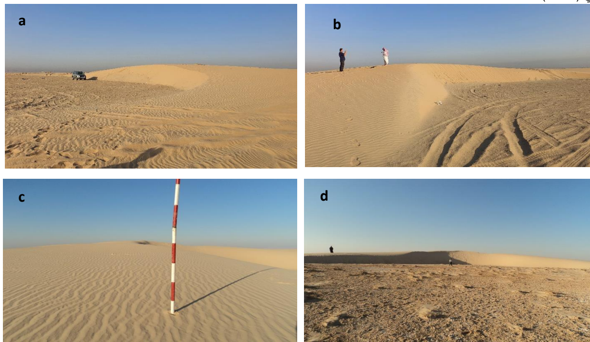
شكل 1. كتبان هلالية في (a, b) شمال شرق الكويت و (c, d) جنوب العراق (النجف).
