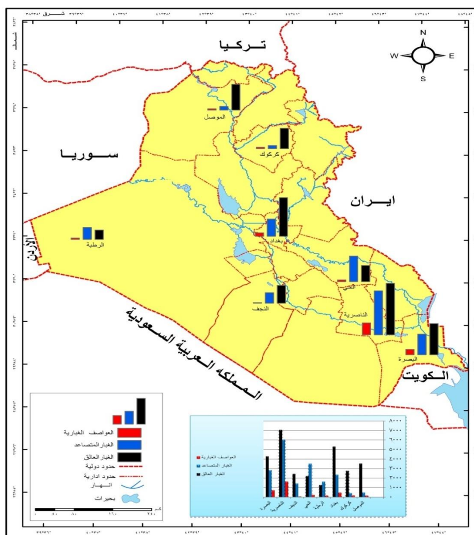
شكل (5) المجموع السنوي لتكرار الظواهر الغبارية في محطات الدراسة . المصدر / عمل الباحثة بالاعتماد على بيانات الجدول (3)
