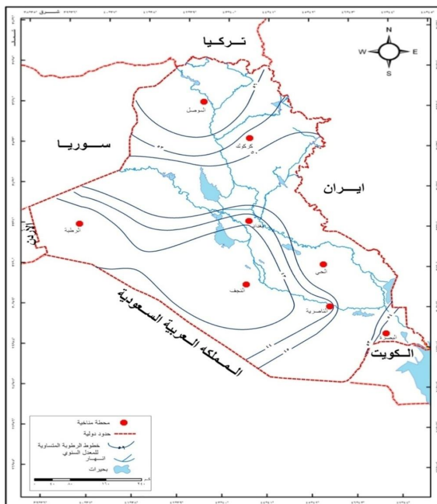
شكل (2) خطوط تساوي المعدلات السنوية للرطوبة النسبية (%) لمحطات الدراسة للمدة (1941 - 2012) . المصدر : عمل الباحثة بالاعتماد الجدول (2) .
