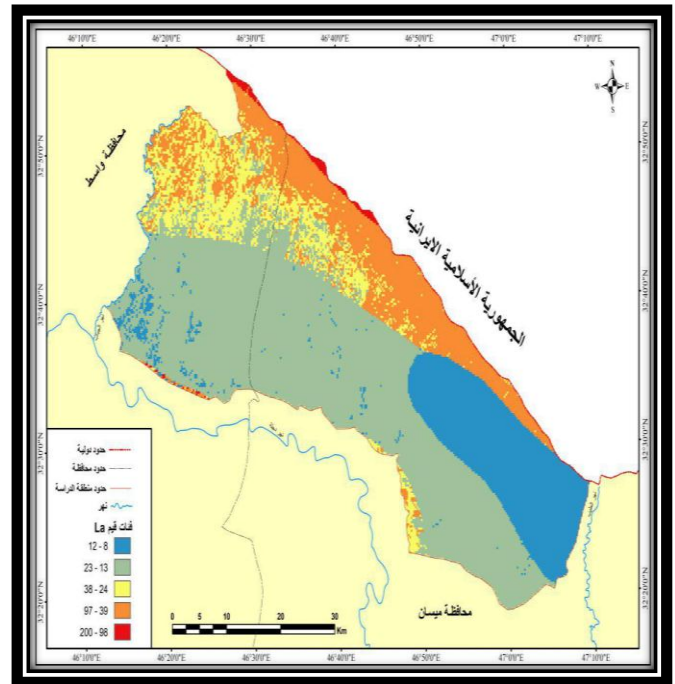
خريطة (6) توزيع قيم (la) لمراوح منطقة الدراسة
