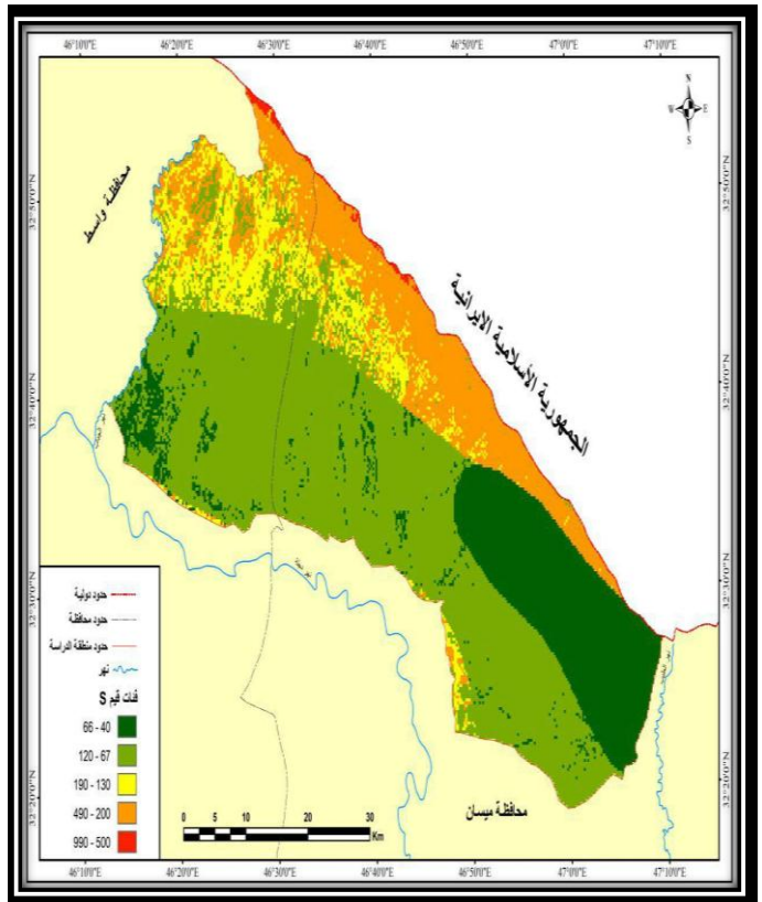
خريطة (5) توزيع قيم ( S ) للمراوح في منطقة الدراسة
