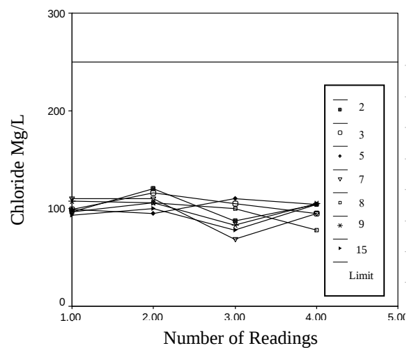
شكل رقم (9) : الكلوريد لماء الشرب للمحطات التي لها أربعة قراءات
