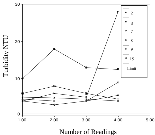
شكل رقم (3) : العكورة لماء الشرب للمحطات التي لها أربعة قراءات
