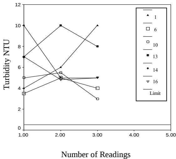
شكل رقم (2) : العكورة لماء الشرب للمحطات التي لها ثلاثة قراءات
