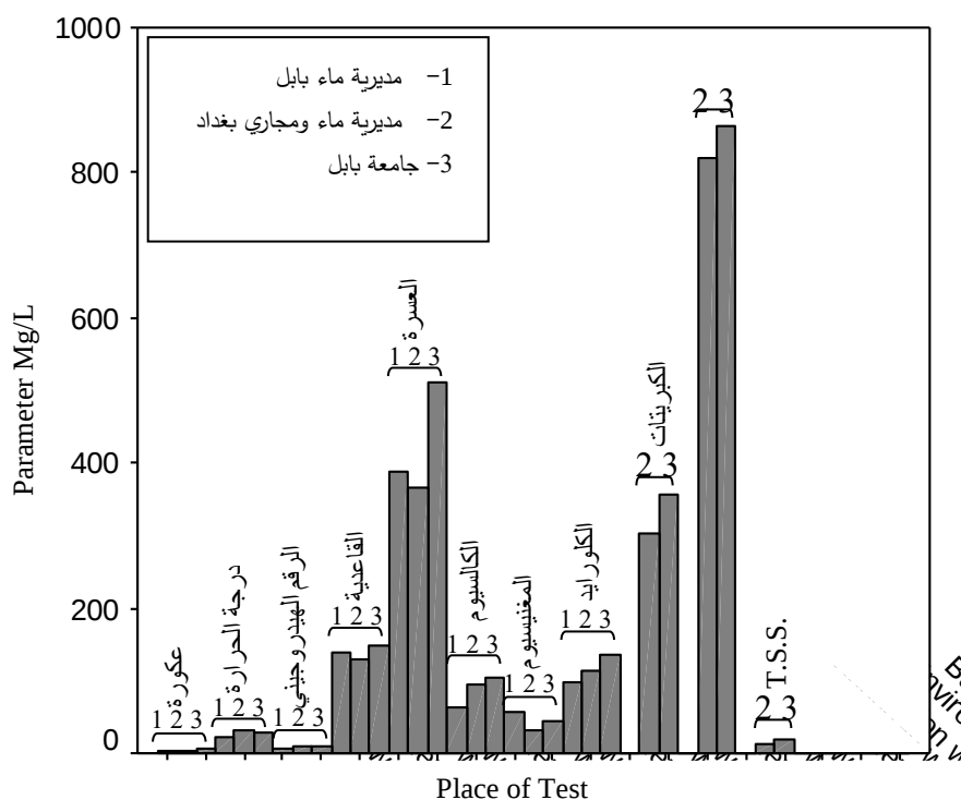
شكل رقم ( 12 ) : مقارنة لنتائج فحص ماء الشرب من قبل كل من مديرية ماء بابل، مديرية ماء ومجاري بغداد، جامعة بابل.
