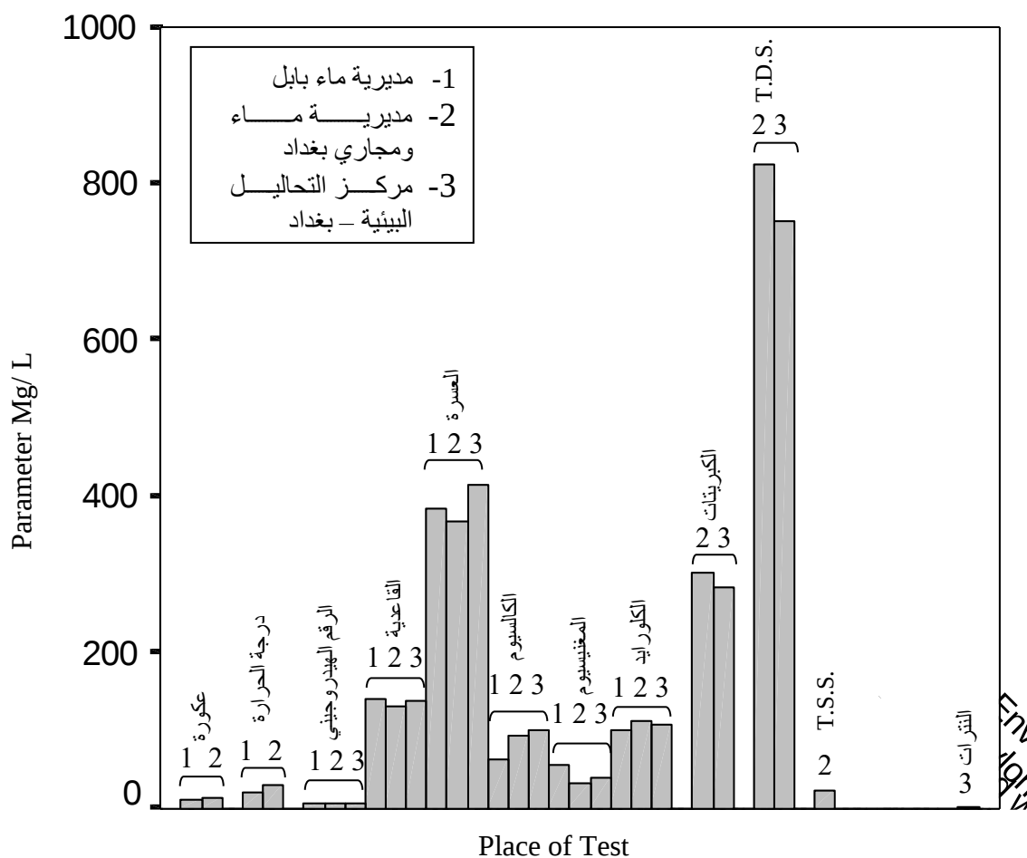
شكل رقم ( 11 ) : مقارنة لنتائج فحص الماء الخام من قبل كل من مديرية ماء بابل، مديرية ماء ومجاري بغداد، ووزارة البيئة / مركز التحاليل البيئية - بغداد
