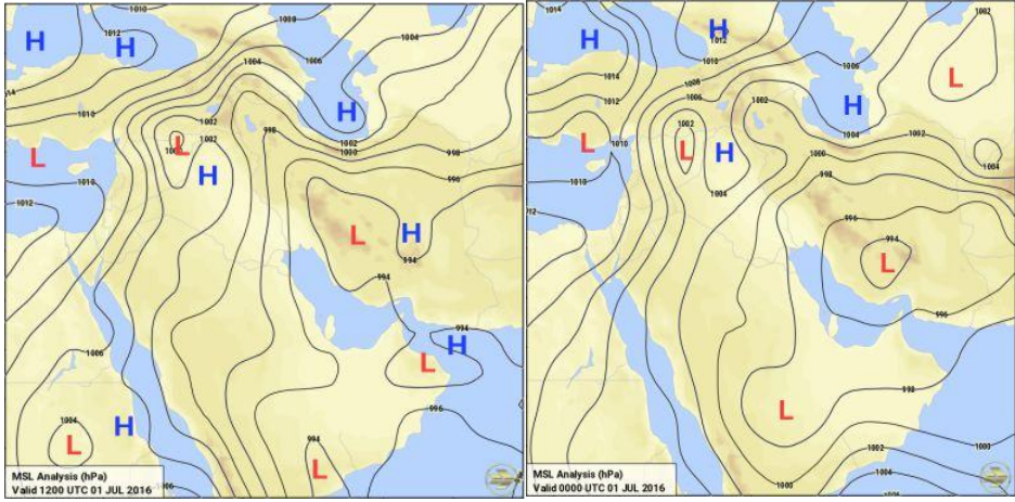
شكل ( ١٤ أ) بداية نهاية موجة الحر باندماج الهندي مع السوداني ، شكل ( ١٤ ب) نهاية الموجة الحارة كلياً نهراً ٢٠١٦/٧/١
