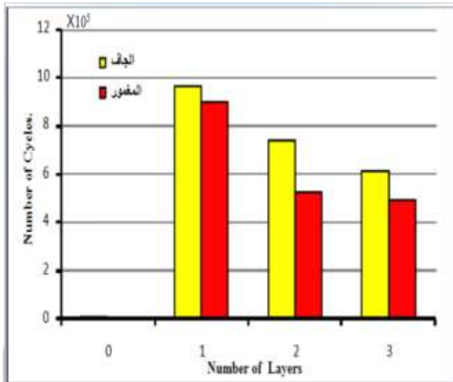
الشكل ( ٢ ) يوضح مقارنة بين عدد دورات الكلال لحد الفشل وعند طبقات التسليح لسترات البوليستر غير المشبع المدعمة بالألياف الزجاجية العشوائية الجافة والمغمورة بالماء
