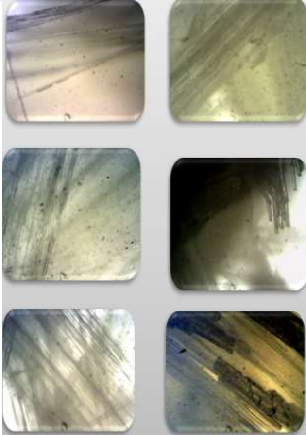
شكل ( 4 ) يوضح الصور المجهرية للعشوائية الجافة والمغمورة بالماء بعد إجراء اختبارات الكلال (10X)
