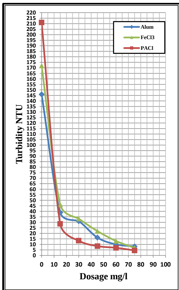
شكل-1: العلاقة بين الجرعة المستخدمة للمخثرات الثلاثة وبين العكارة عند مستوى عكارة (580 NTU)
