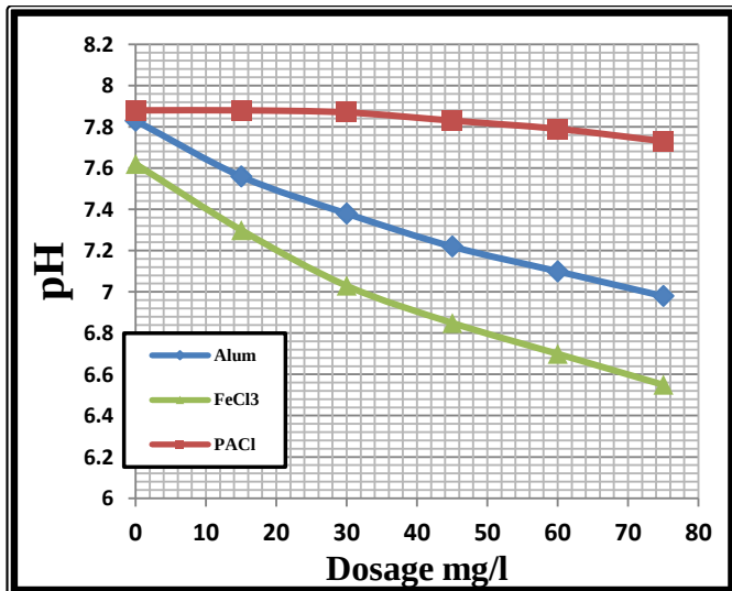
شكل-4: العلاقة بين الجرعة المستخدمة للمخثرات الثلاث ومقدار الـ pH عند مستوى العكارة (52 NTU)
