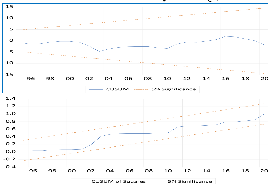
الشكل (١): اختبار الاستقرار الهيكلي لأنموذج معدل النمو الاقتصادي
