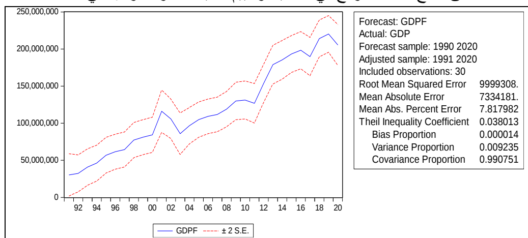
الشكل (٢): القيم الفعلية والمقدرة لأنموذج معدل النمو الاقتصادي
