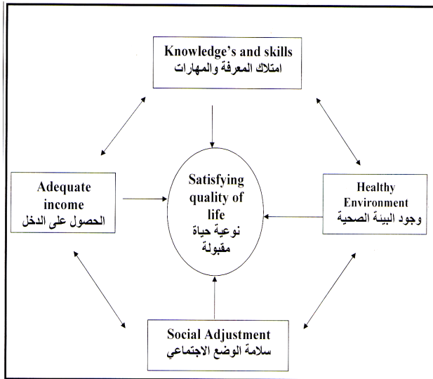
الشكل رقم (1) يوضح طبيعة العلاقة بين متطلبات نوعية الحياة المقبولة (١).
