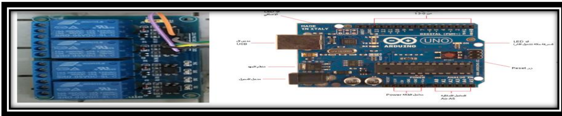
شكل (1) الدائرة الإلكترونية الخاصة بتشغيل الجهاز
