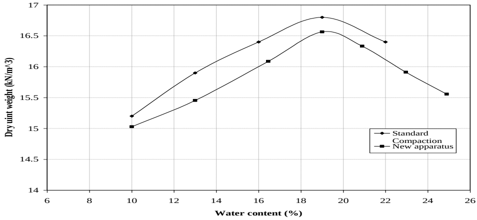
شكل (10): مقارنة بين نتائج الرص لتربة موقع في الكوت.
