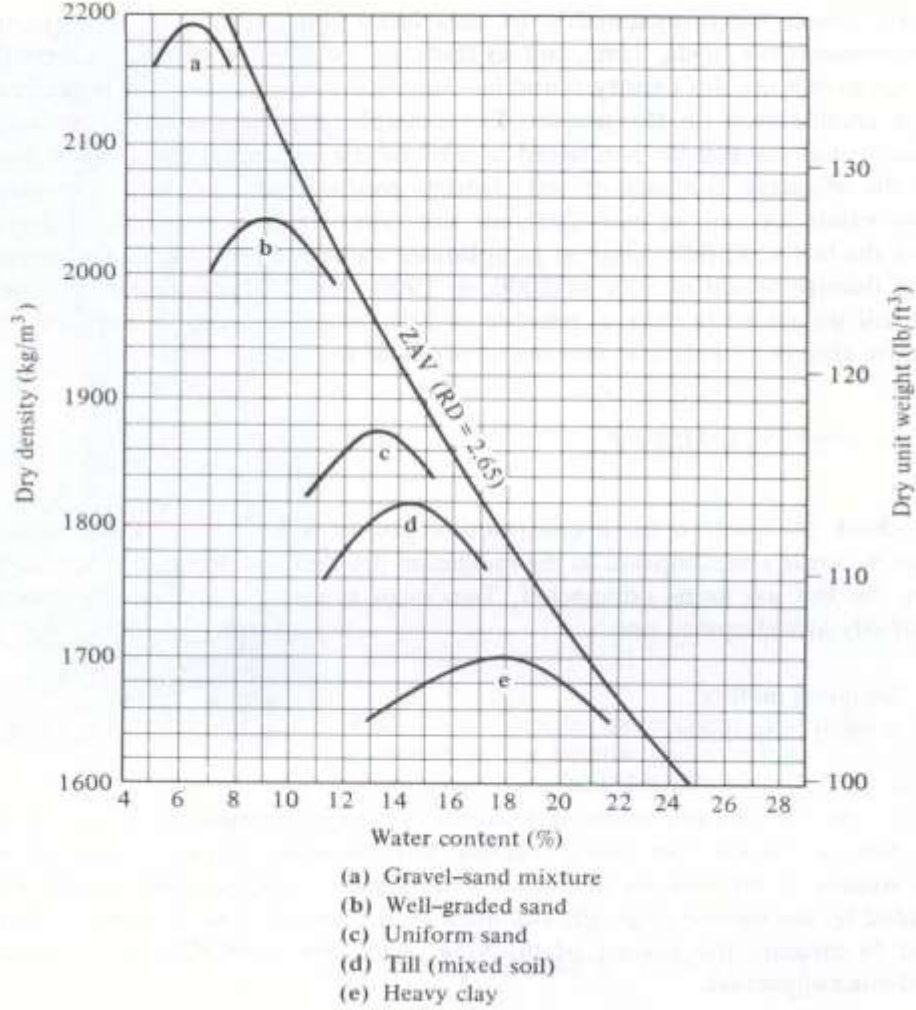
الشكل (٣): منحنيات الرص لأنواع مختلفة من التربة
