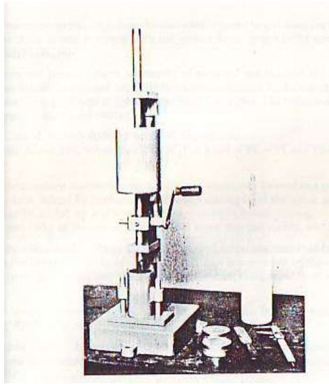
شكل رقم (٥) : تفاصيل الرص بجهاز Dietert.
