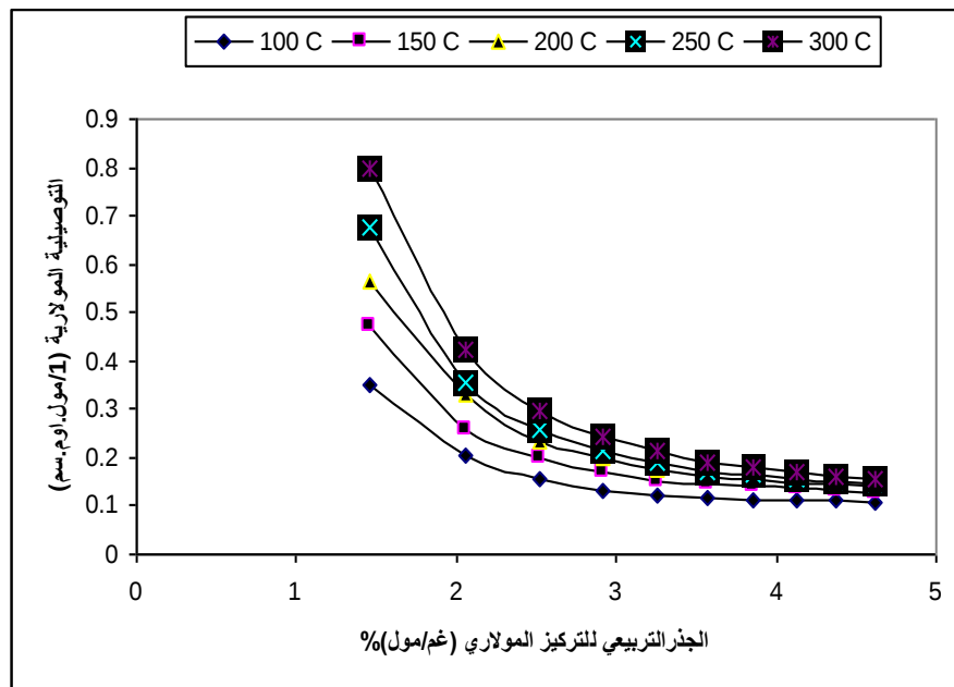
الشكل (4) يوضح العلاقة بين التوصيلية المولارية والجذر التربيعي للتركيز المولاري بعد اضافة اسود الكربون
