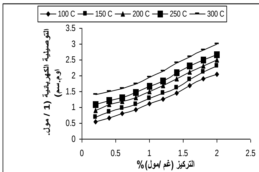
الشكل (1) يوضح العلاقة بين التوصيلية الكهربائية والتركيز قبل اضافة اسود الكربون
