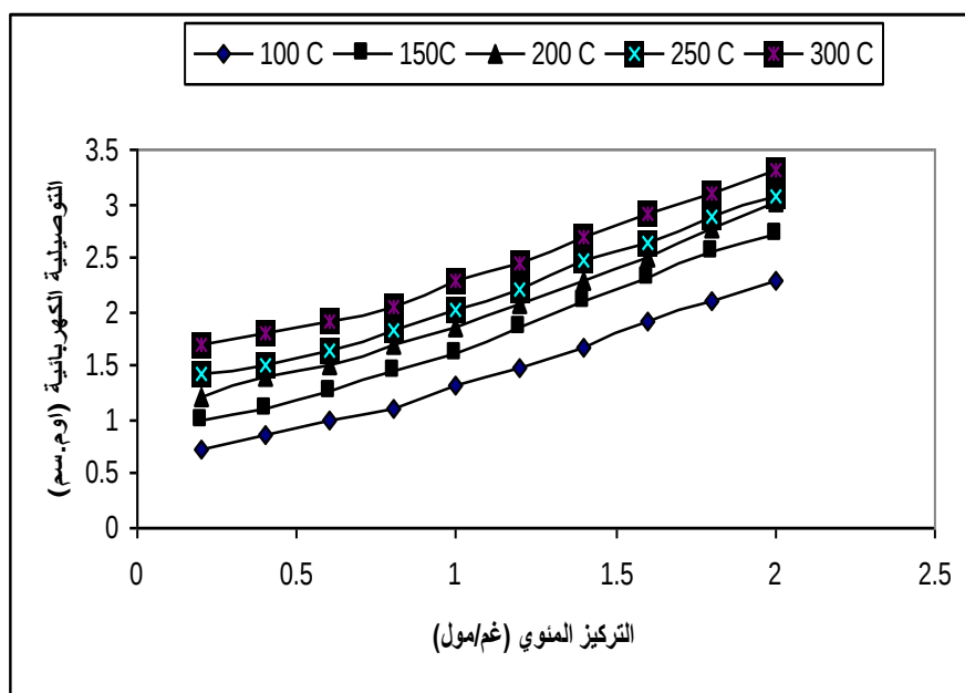
الشكل (2) يوضح العلاقة بين التوصيلية الكهربائية والتركيز بعد اضافة اسود الكربون
