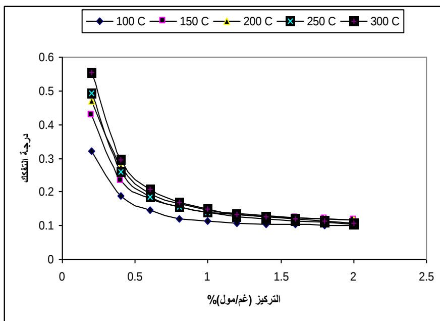
الشكل (6) يوضح العلاقة بين درجة التفتك والتركيز المئوي بعد اضافة اسود الكربون
