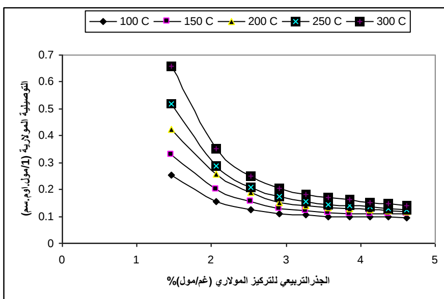
الشكل (3) يوضح العلاقة بين التوصيلية المولارية والجذر التربيعي للتركيز قبل اضافة اسود الكربون
