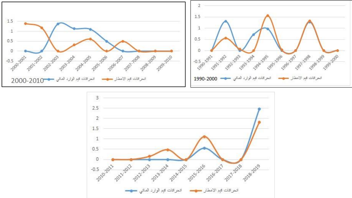
شكل (٢) انحرافات قيم الوارد المائي ومعدلات الامطار عن معدلاتها أثناء المدة ١٩٩٠-٢٠١٩
