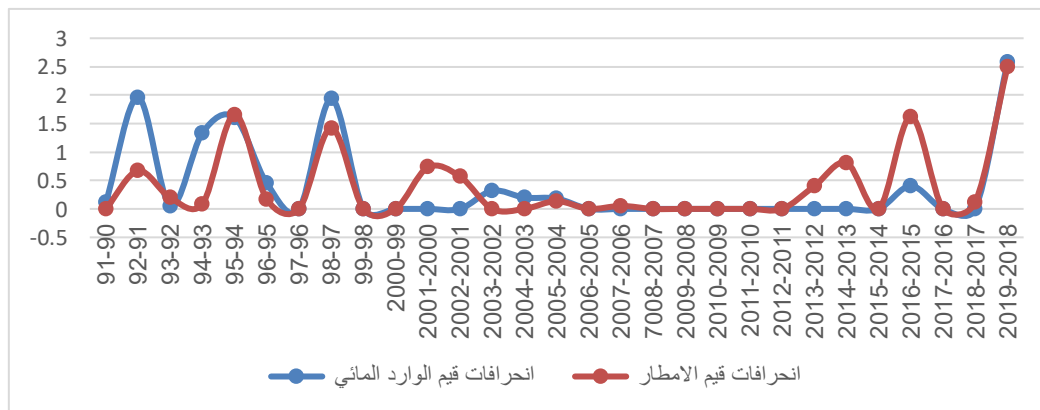
شكل (١) انحرافات قيم الوارد المائي ومعدلات الامطار عن معدلاتها أثناء المدة ١٩٩٠-٢٠١٩
