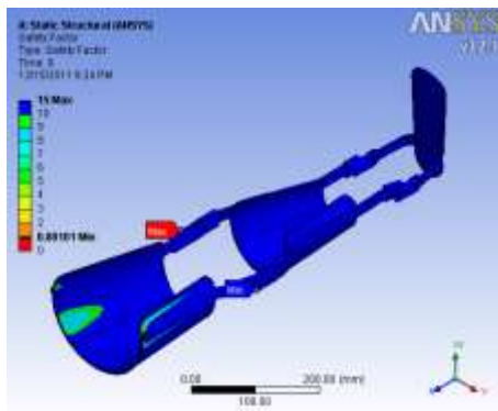
A: Polypropylene KAFO
