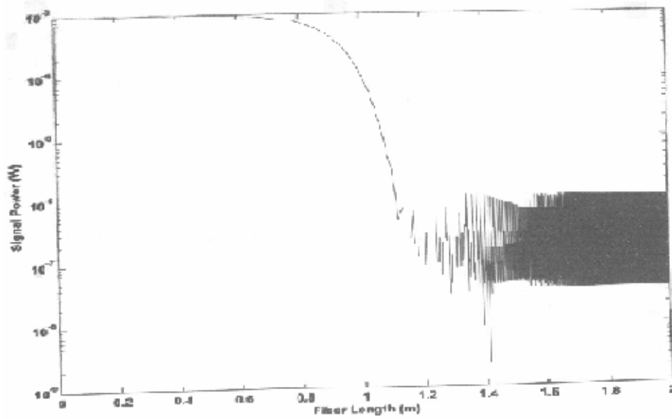
شكل رقم ( 7 ) : يمثل العلاقة بين قدرة الإشارة الداخلة الى المكبر وطول الليف الضوئي لاي تجاوز 2M
