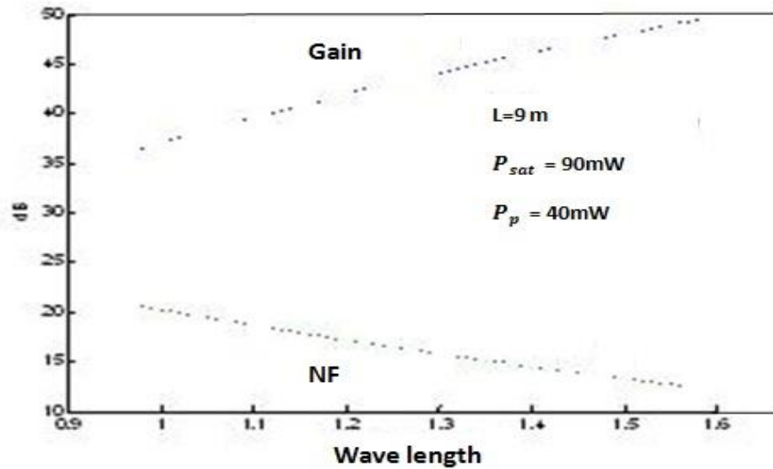
شكل رقم (5) : العلاقة بين الكسب وعامل الضوضاء كدالة لطول موجة الضخ ولطول (9m). ويتبين من هذه النتائج بأن طول الليف المكبر يجب أن لا يقل عن ( 9m ) ، وهذا ينطبق مع معظم نتائج البحوث المنشورة التي يكون فيه طول الليف الضوئي المكبر دائماً بحدود 13m أو أكثر [15].
