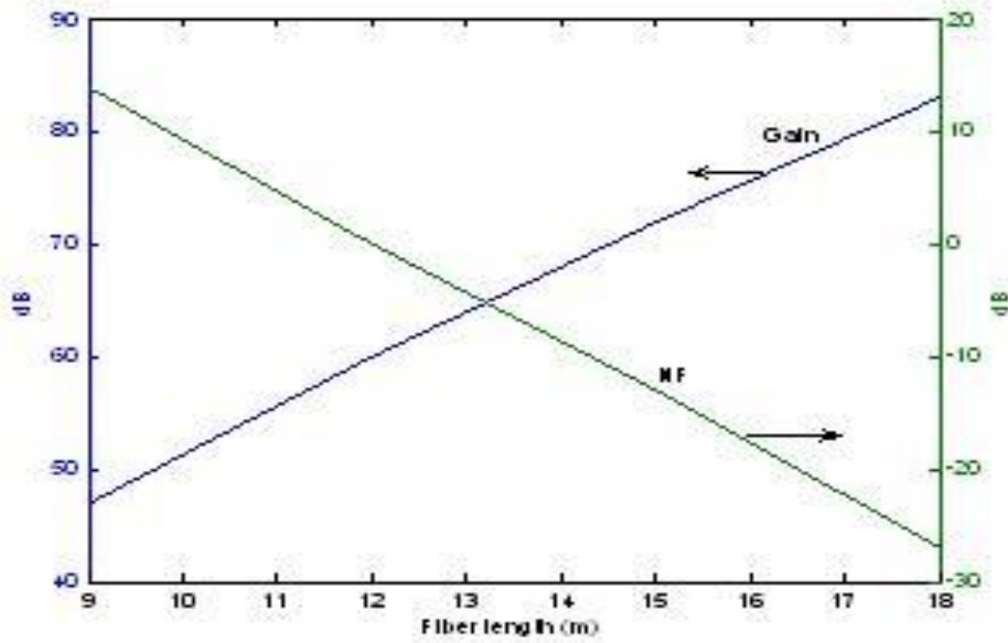
شكل رقم (6): العلاقة بين الكسب وعامل الضوضاء كدالة لطول الليف الضوئي المكبر
