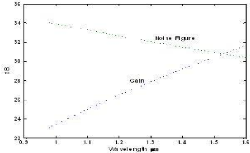
شكل رقم (4): العلاقة بين الكسب وعامل الضوضاء كدالة لطول موجة الضخ ولطول (6m).
