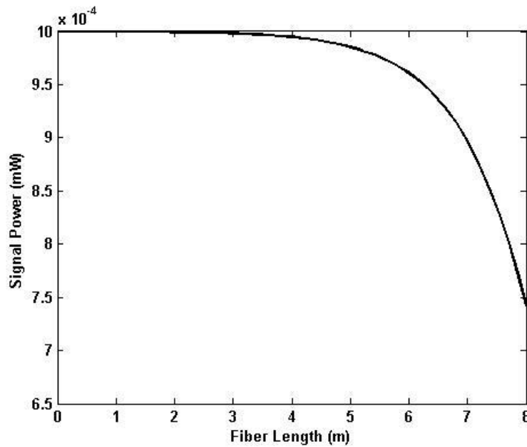
شكل رقم (8) : يمثل العلاقة بين قدرة الإشارة الداخلة الى المكبر وطول الليف الضوئي يمتد الى 8M
