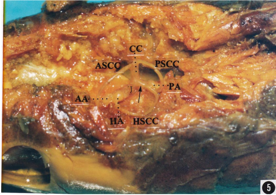
شكل(5): منظر سطحي لتجويف قحف سمكة الخشني يوضح درجة ميل القناة النصف دائرية الافقية وارتباط نهايتها الخلفية بالجزء الخلفي للقريبة (←).
