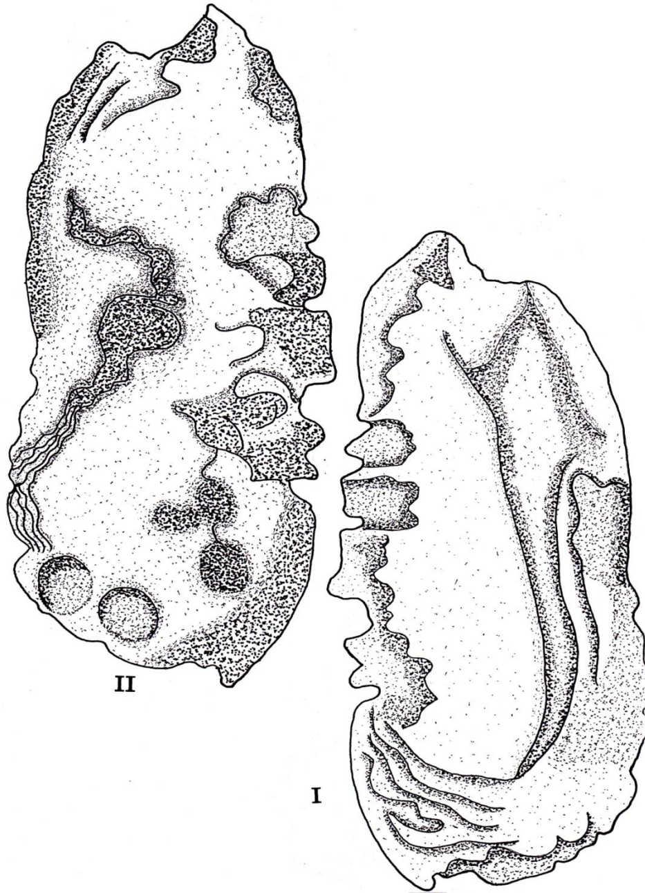
شكل (8): رسم تخطيطي لحصوة الكبيس (السهم Sagitta) في سمكة الخشني (16X).
